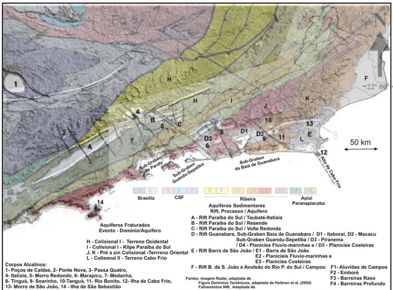
Figura 1 - Mapa dos aquíferos do estado do Rio de Janeiro.
