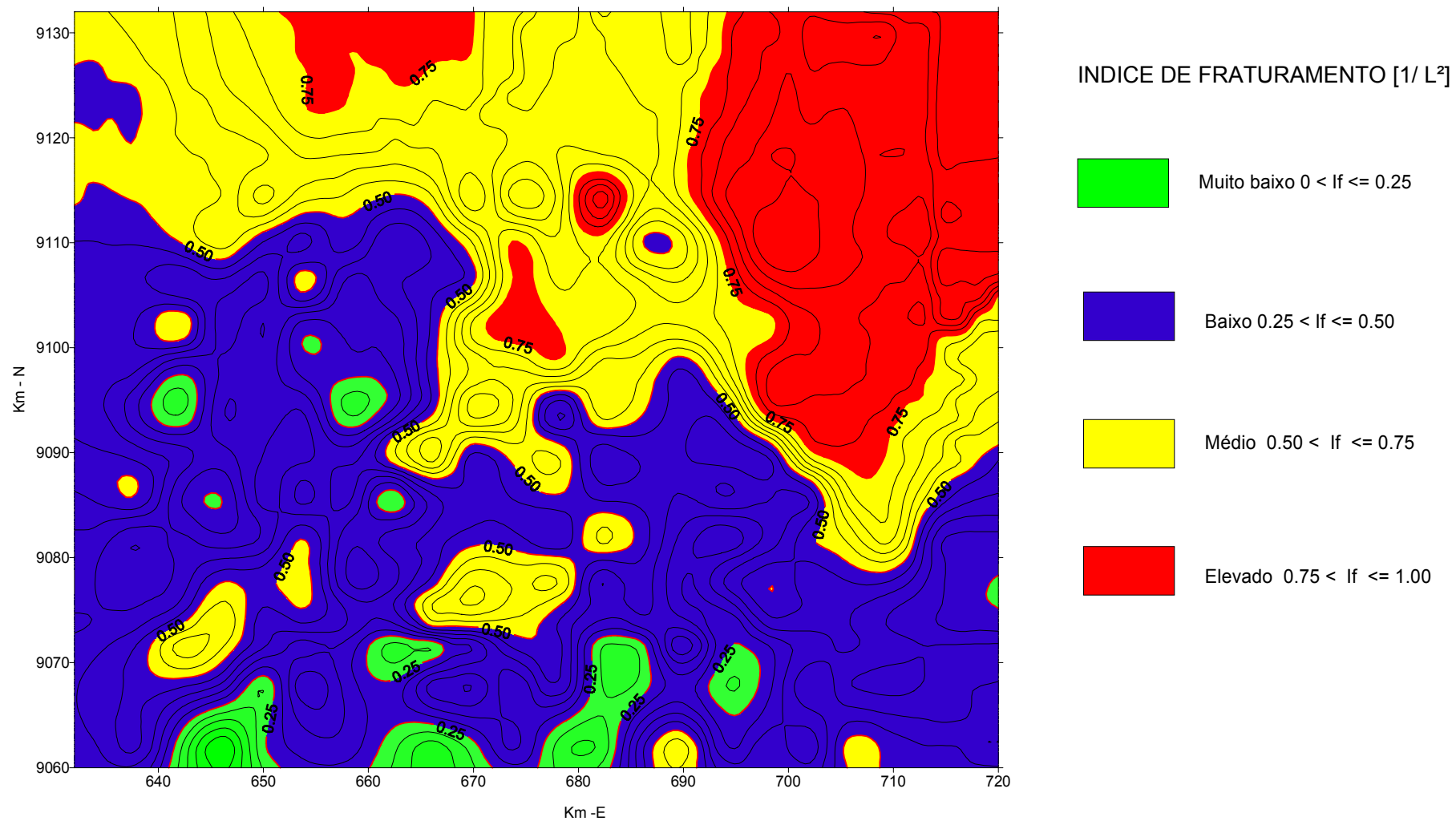
Figura 4.12 – Mapa de índices de fraturamento do cristalino indiferenciado do Alto Moxotó
