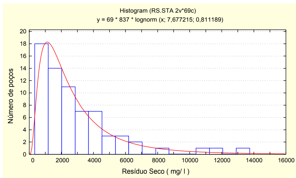
Figura 4.13 – Distribuição de probabilidade log-normal do resíduo seco das águas subterrâneas do cristalino indiferenciado do Alto Vale do Rio Moxotó –PE.
