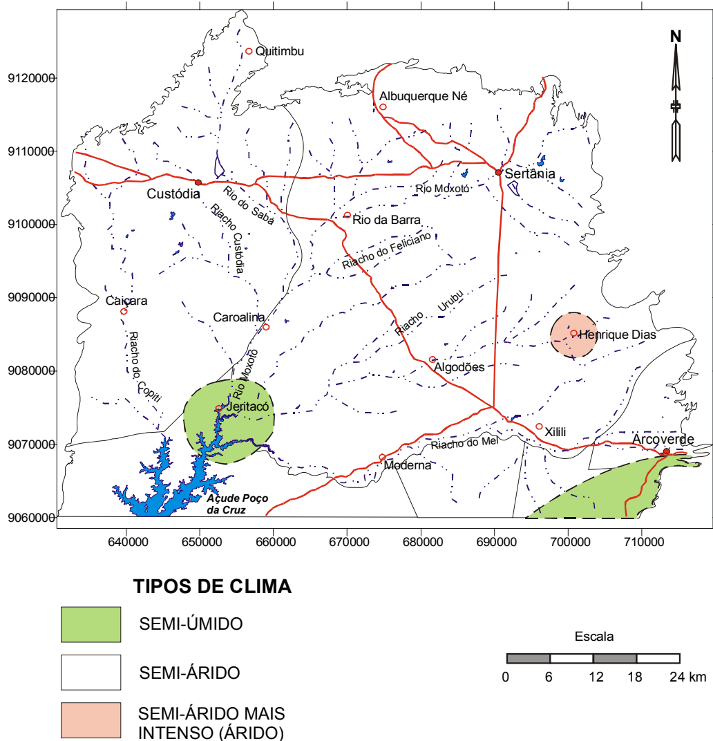
Figura 2.5. Mapa climático da área do Alto Vale do Rio Moxotó.
