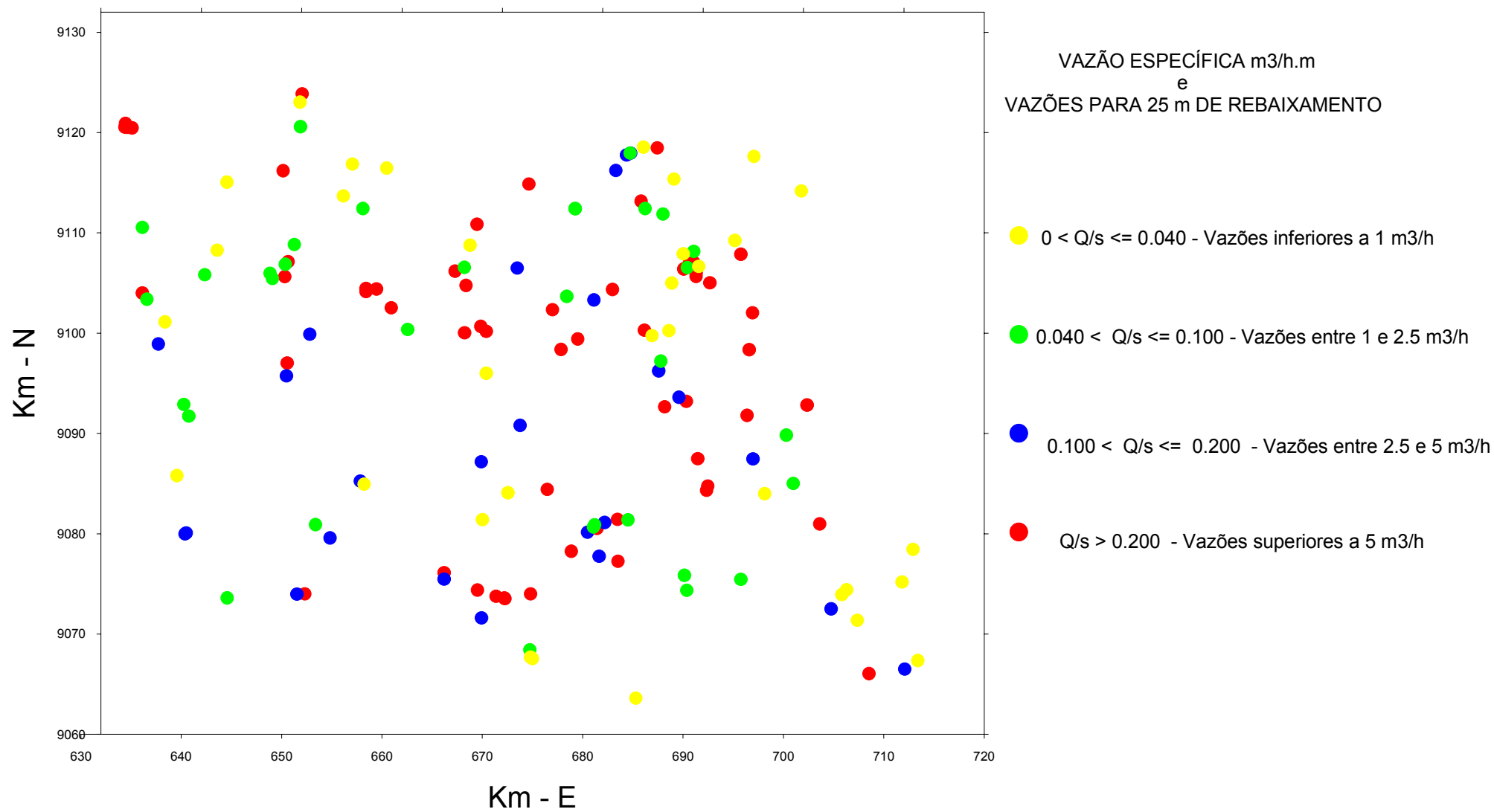
Figura 4.10 – Mapa de valores pontuais de vazão específica e vazões para 25 m de rebaixamento nos poços do cristalino indiferenciado do Alto Moxotó.
