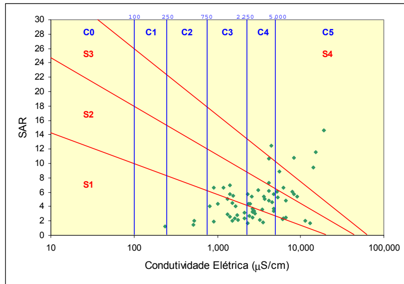
Figura 4.18 - Classificação da água das rochas cristalinas para a irrigação, segundo o U.S. Salinity Laboratory (apud Logan, 1965).
