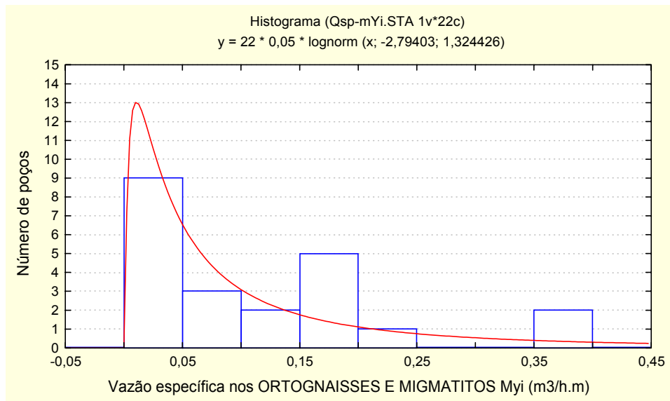
Figura 4.8 – Distribuição de probabilidade da vazão específica dos poços os ORTOGNAISSES e MIGMATITOS.- MYi.
