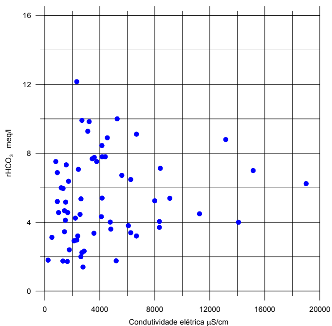
Figura 4.16 – Gráfico de dispersão de pontos, mostrando a falta de correlação entre a condutividade elétrica e o íon bicarbonato, das águas subterrâneas do cristalino indiferenciado do Alto Moxotó.
