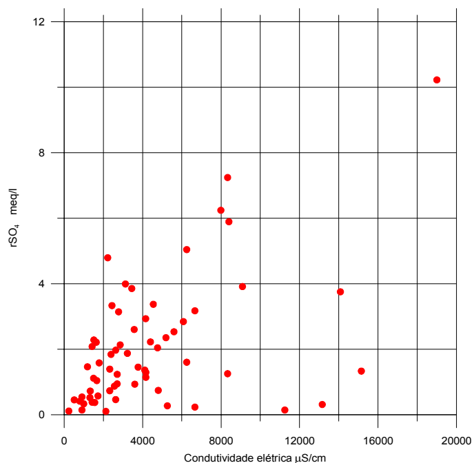
Figura 4.17 – Gráfico de dispersão de pontos, mostrando a falta de correlação entre a condutividade elétrica e o íon sulfato, das águas subterrâneas do cristalino indiferenciado do Alto Moxotó.
