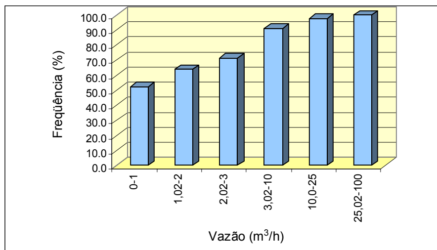
Figura 4.6. Histogramas de vazões de poços para tempo de bombeamento de 12 horas. (a) Frequência, (b) Frequência Acumulada.
