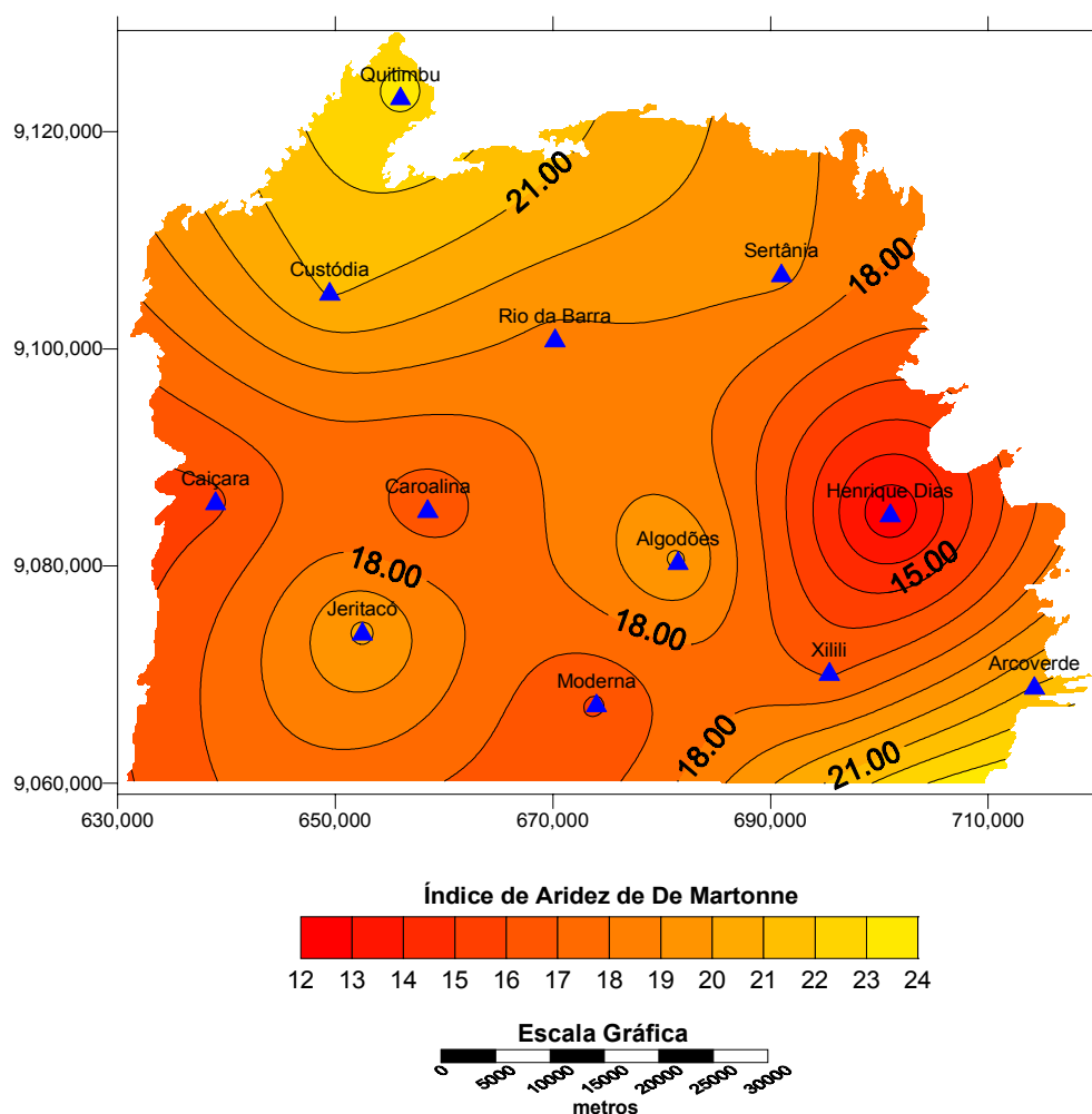
Figura 2.4 – Mapa de aridez segundo E. De Martonne.
