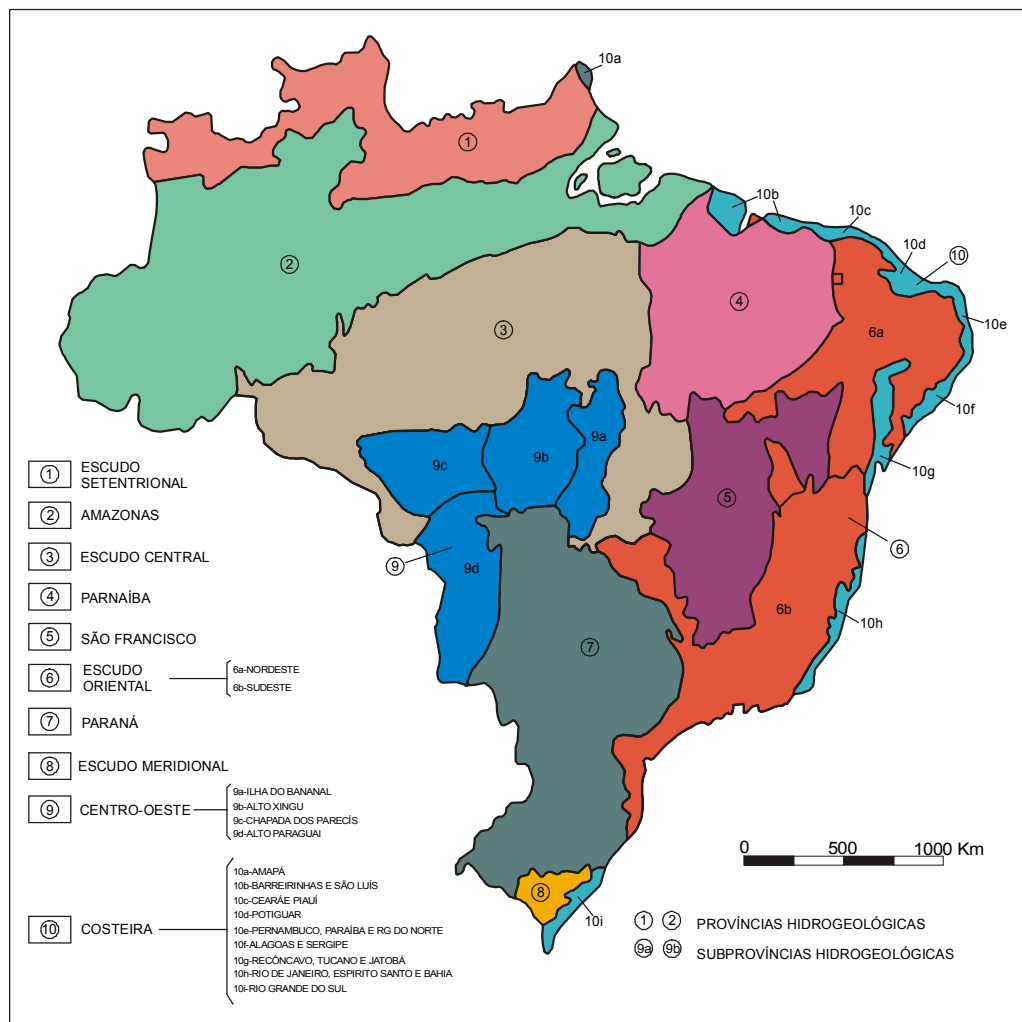
Figura 4.1. Províncias e Subprovíncias Hidrogeológicas do Brasil.
