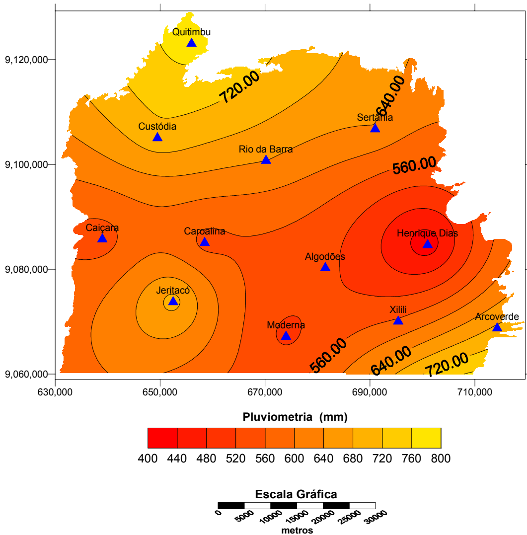
Figura 2.1. Mapa de isoietas da área do Alto Vale do Rio Moxotó.
