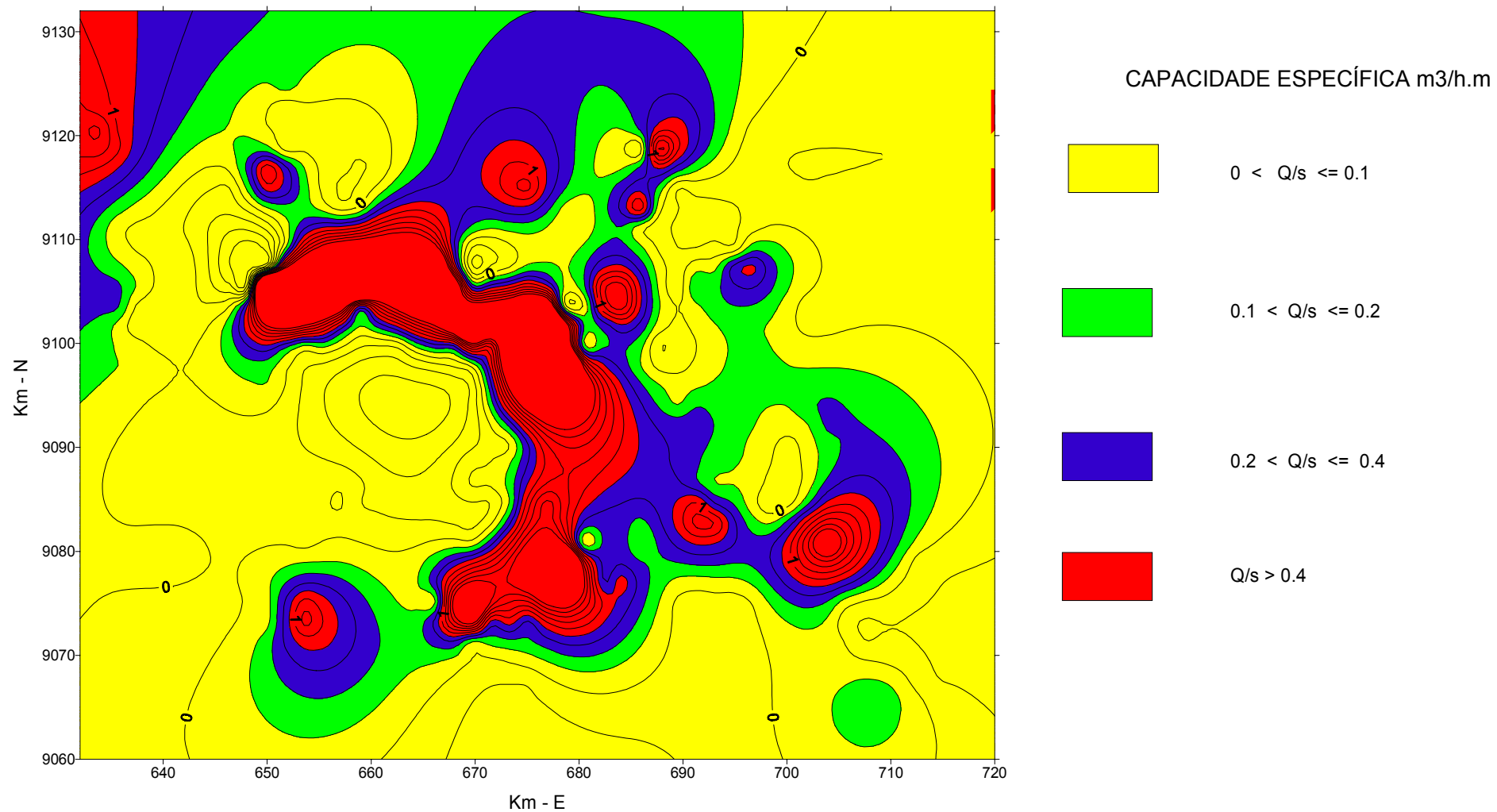
Figura. 4.11 – Mapa de capacidade específica dos poços do cristalino indiferenciado da área do Alto Moxotó.
