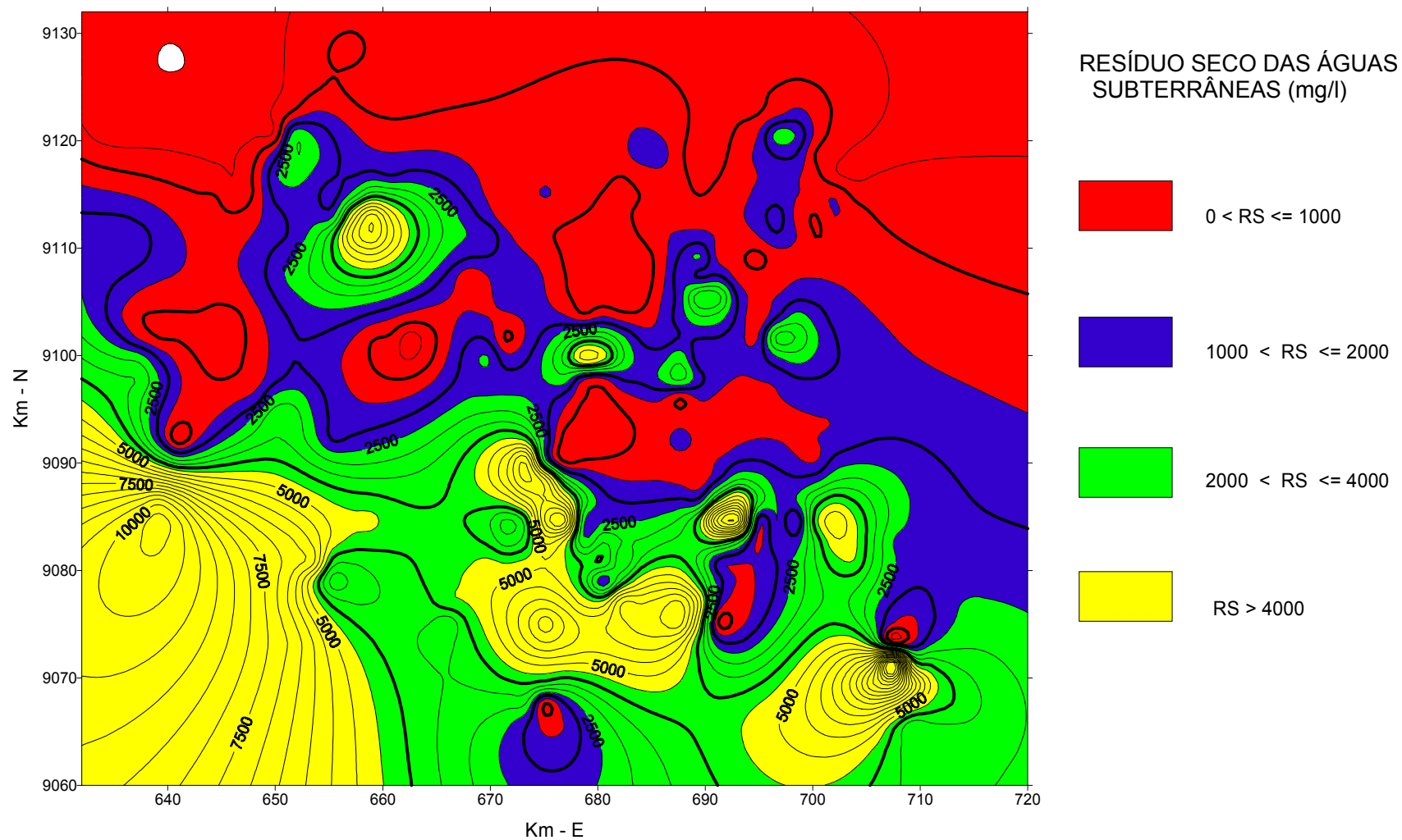
Figura 4.19 – Mapa de residuo seco (mg/l) das águas subterrâneas do cristalino indiferenciado do Alto Moxotó - PE
