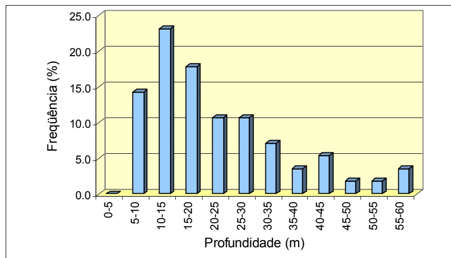
Figura 4.4. Histogramas de profundidade das fendas.
