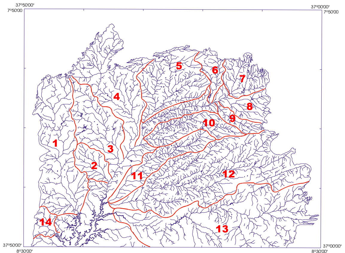
Figura 2.6. Mapa de sub-bacias hidrográficas do Alto Vale do Rio Moxotó.
