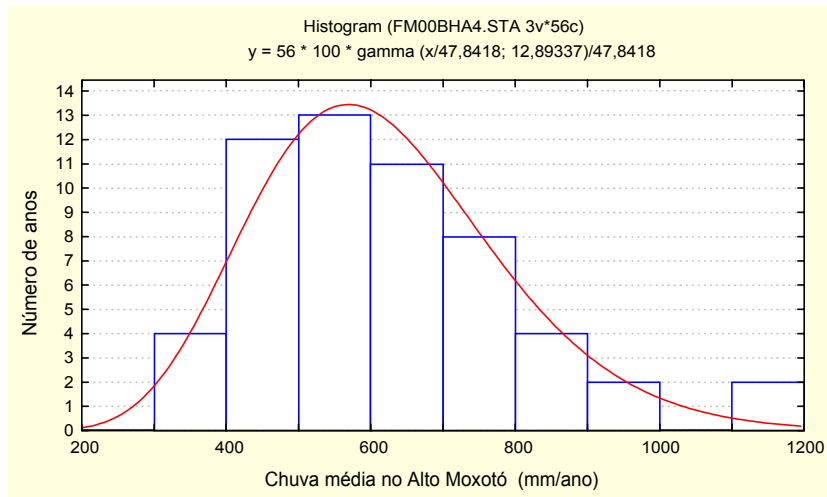
Figura 2.3 – Distribuição gama de probabilidade das chuvas anuais na região do Alto Moxotó.
