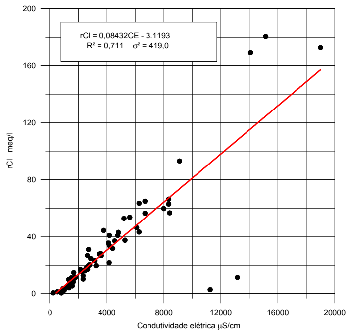
Figura 4. 15 - Gráfico de regressão linear entre a condutividade elétrica e o íon cloreto das águas subterrâneas dos poços do cristalino indiferenciado do Alto Moxotó –PE.
