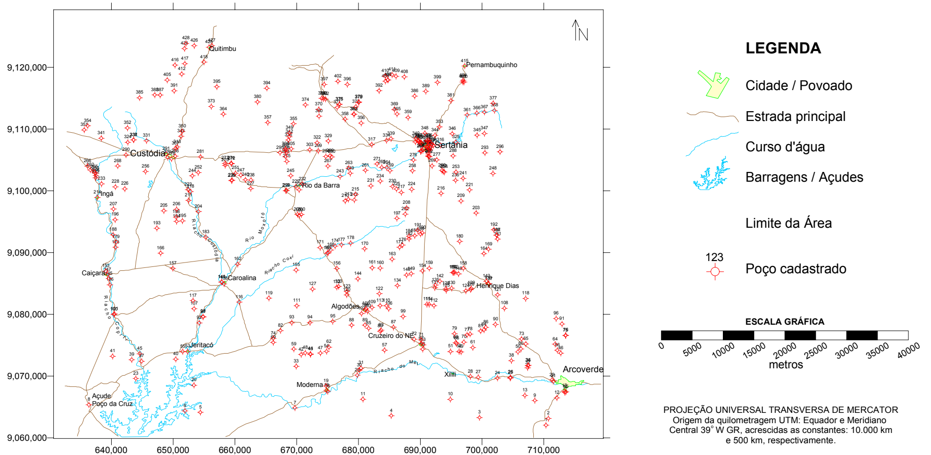
Figura 4.2. Mapa de localização dos poços no Alto Vale do Rio Moxotó.
