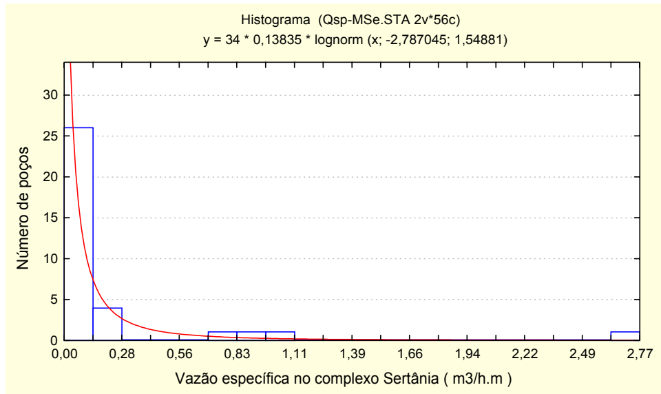
Figura 4.7 – Distribuição de probabilidade da vazão específica dos poços no complexo Sertânia.
