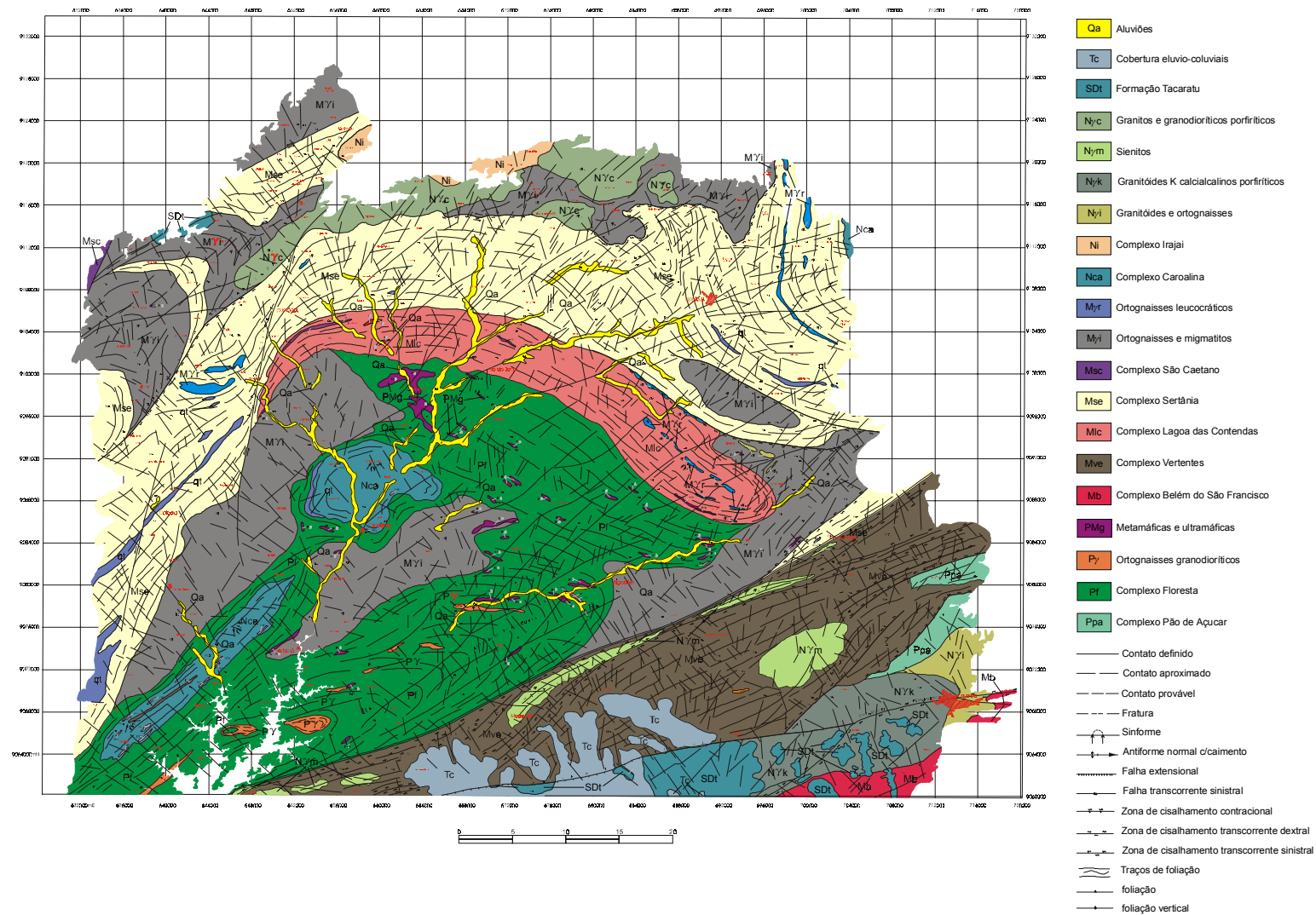
Figura 3.1. Mapa Geológico do Alto Vale do Rio Moxotó.
