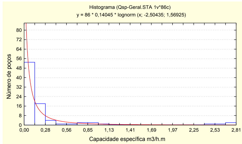
Figura 4.5 – Distribuição de probabilidade log-normal da capacidade específica dos poços do cristalino indiferenciado.
