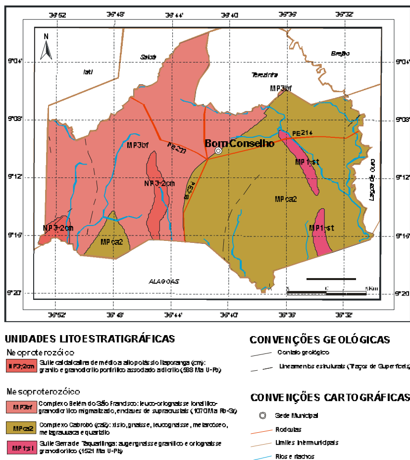
Figura 3 – Mapa geológico
