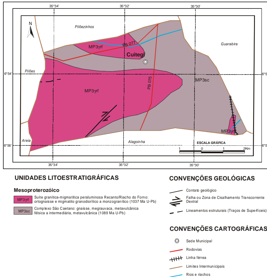
Figura 3 – Mapa Geológico
