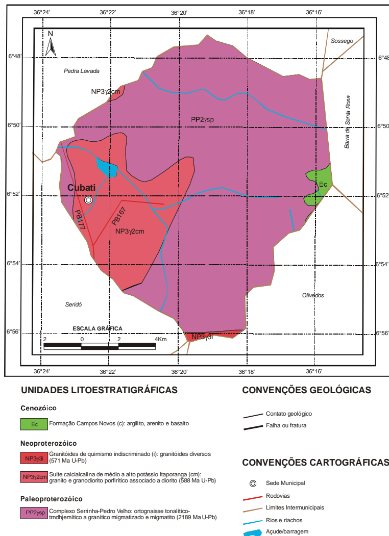
Figura 3 – Mapa Geológico
