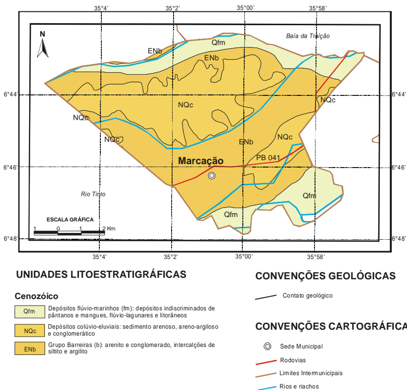
Figura 3 – Mapa Geológico
