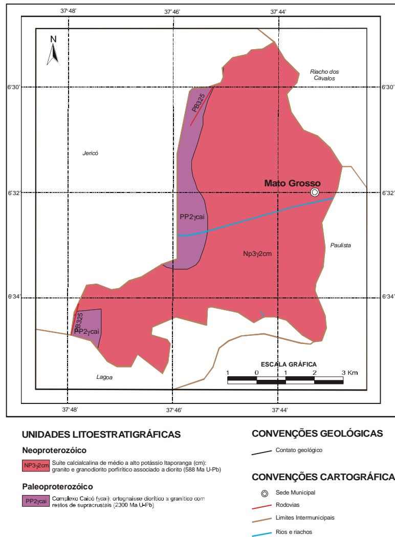
Figura 3 – Mapa Geológico
