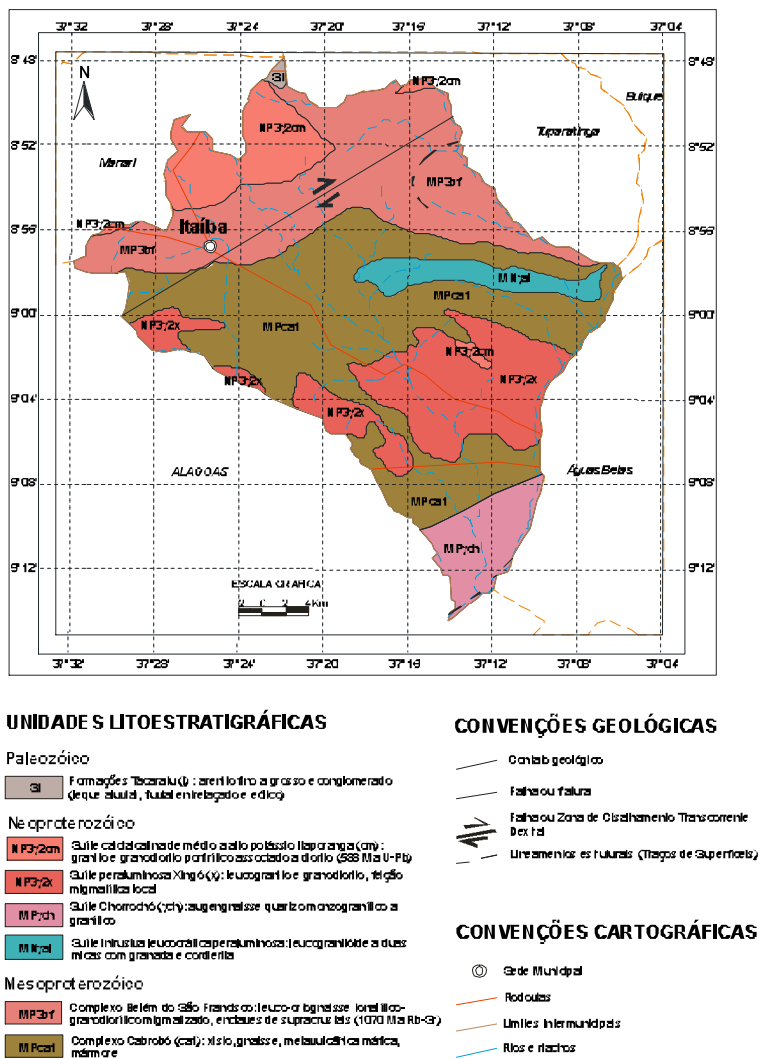
Figura 3- Mapa Geológico
