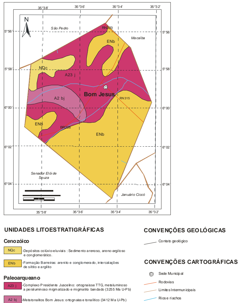
Figura 3 - Mapa Geológico
