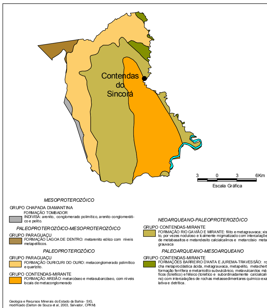
Figura 3 – Esboço geológico.
