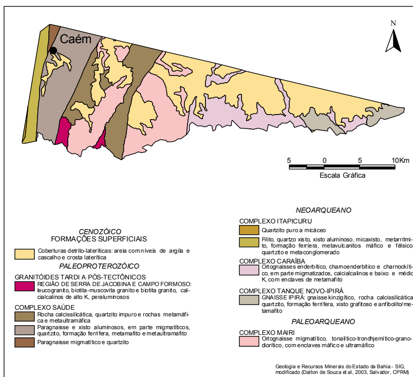
Figura 3 – Esboço geológico.
