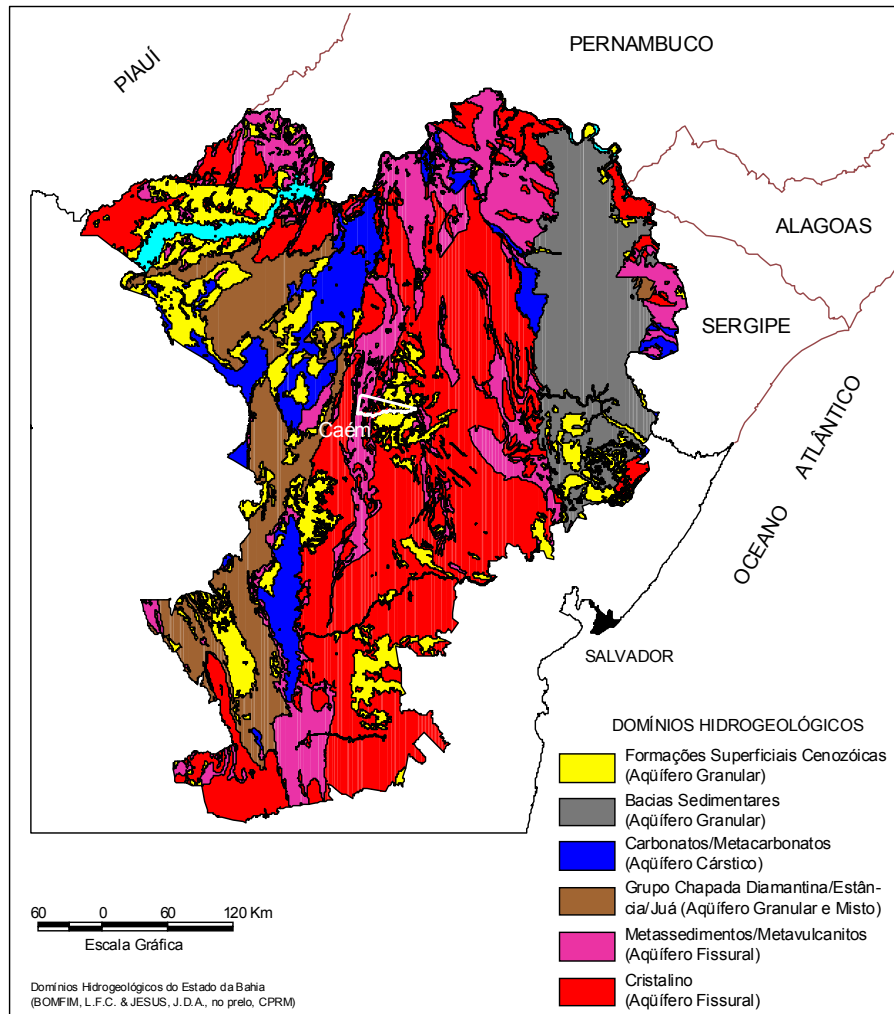
Figura 4 – Domínio hidrogeológico.
