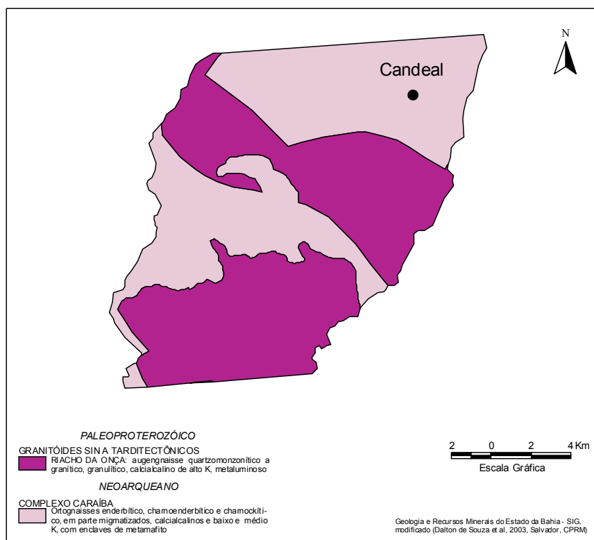
Figura 3 – Esboço geológico.
