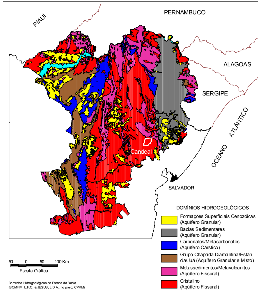
Figura 4 – Domínio hidrogeológico.
