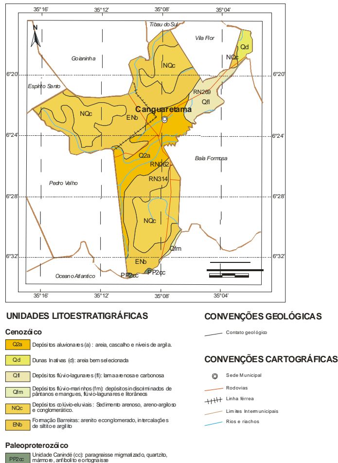
Figura 3 - Mapa Geológico
