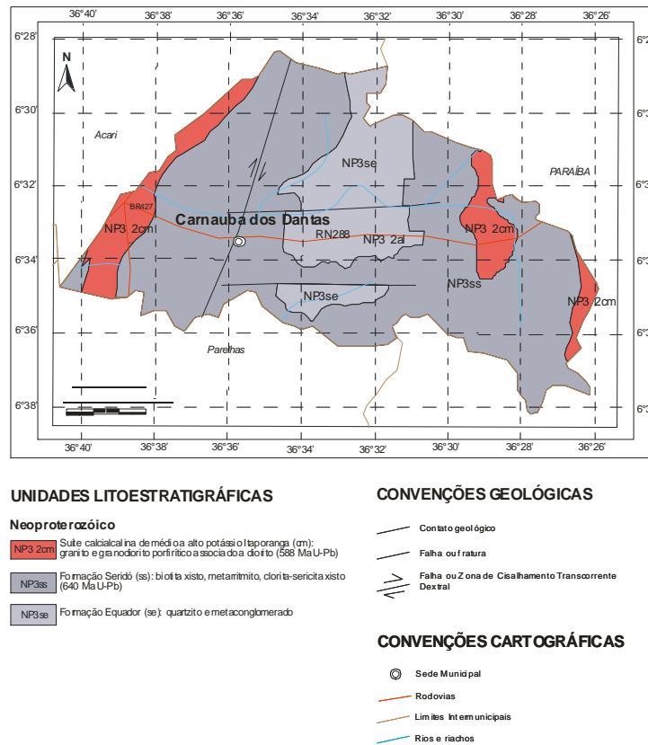
Figura 3 - Mapa Geológico
