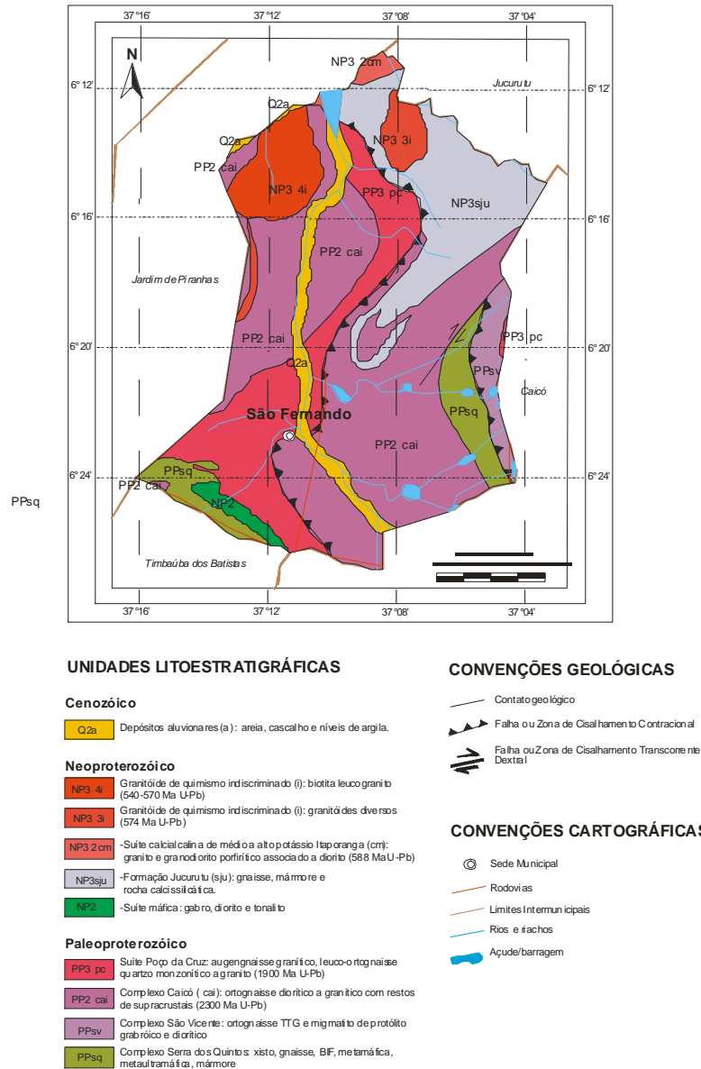
Figura 3 - Mapa Geológico
