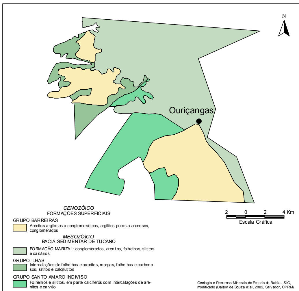
Figura 3 – Esboço geológico.
