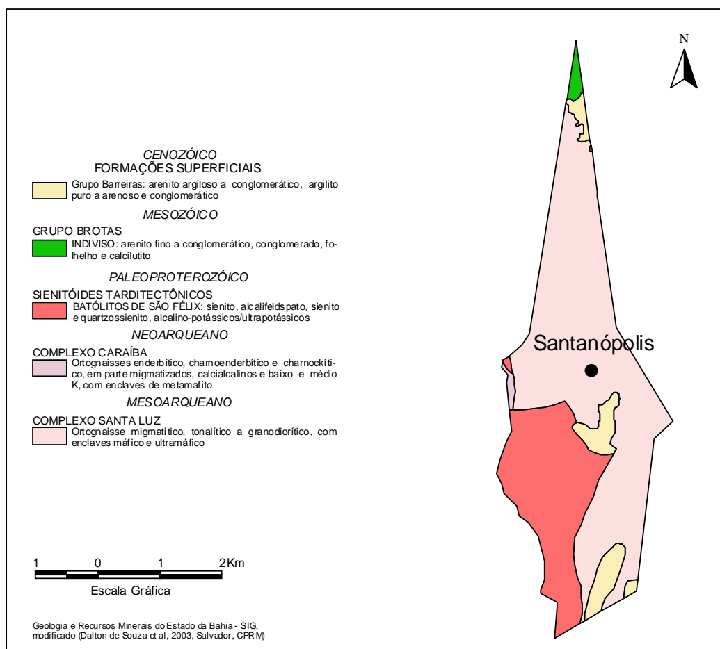
Figura 3 – Esboço geológico.
