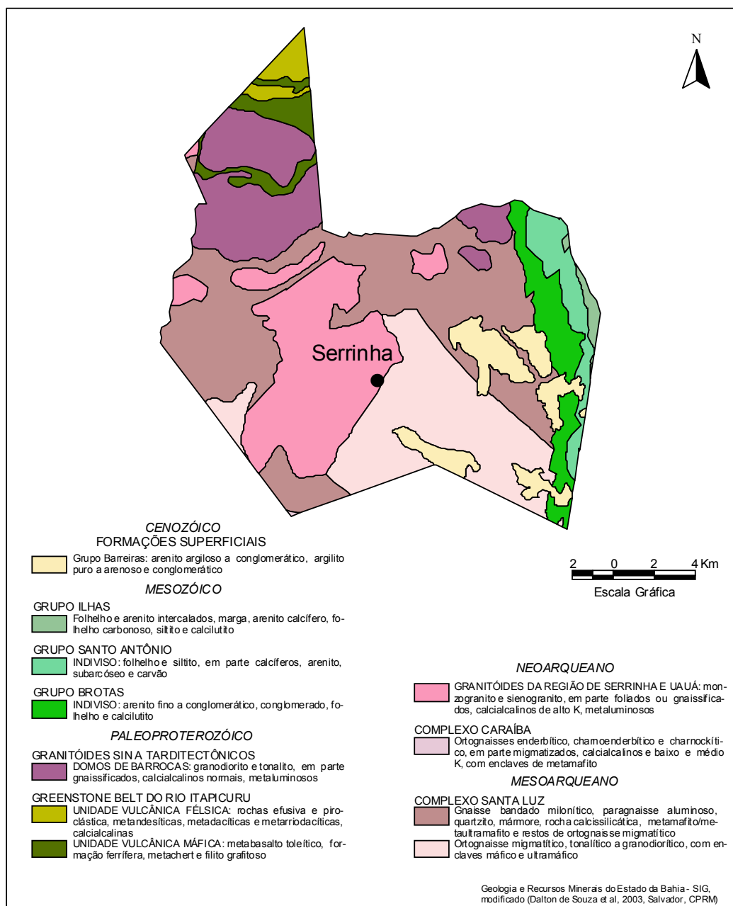
Figura 3 – Esboço geológico.
