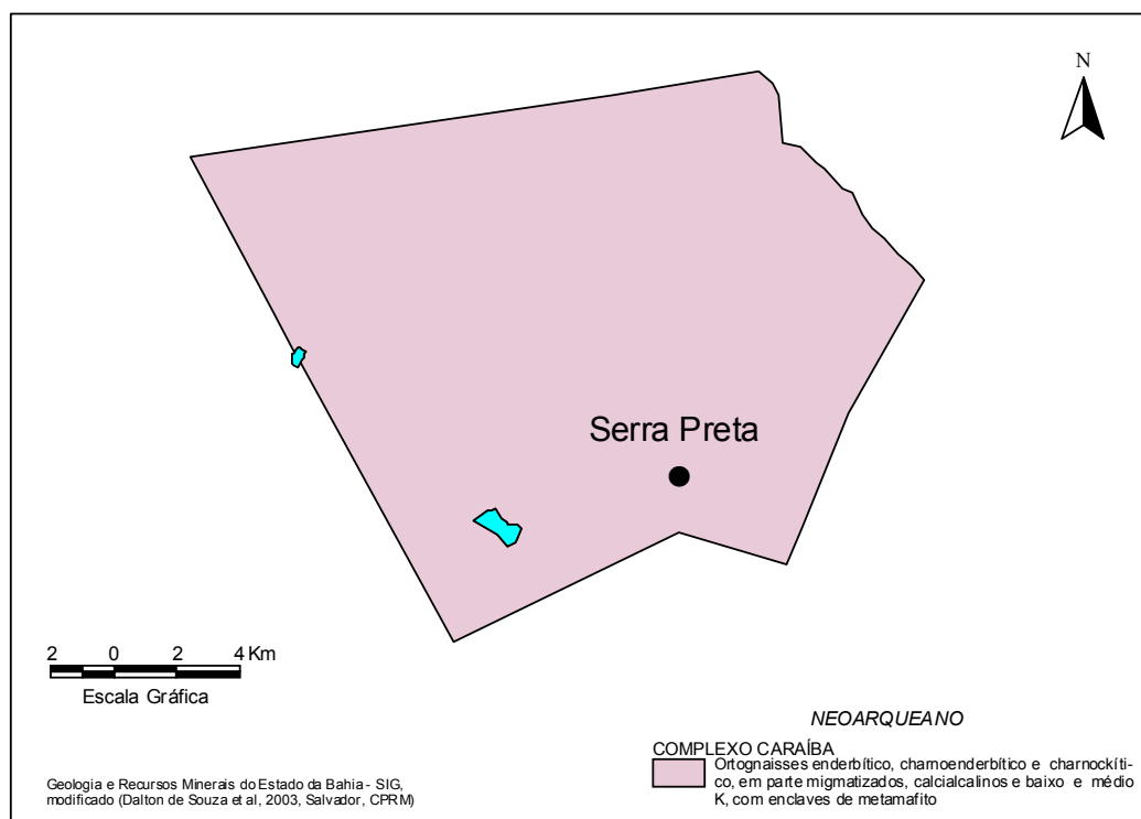
Figura 3 – Esboço geológico.
