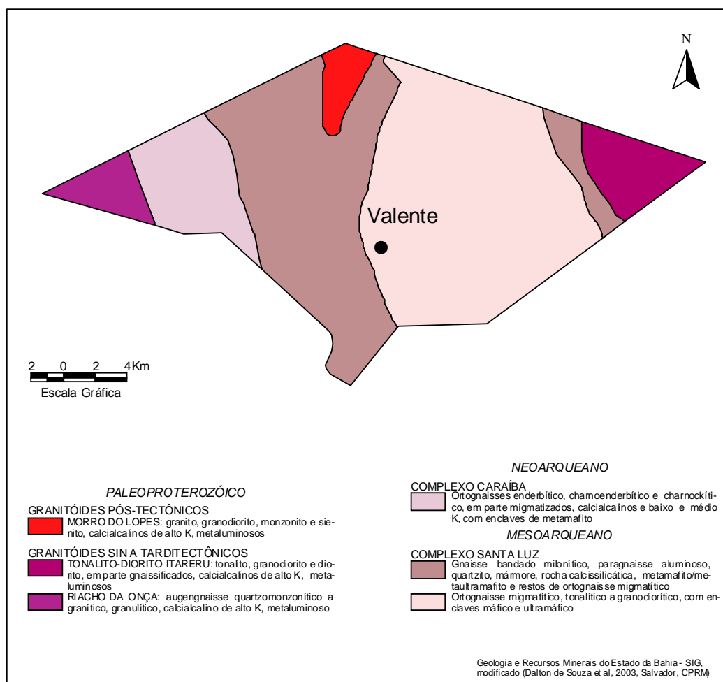
Figura 3 – Esboço geológico.
