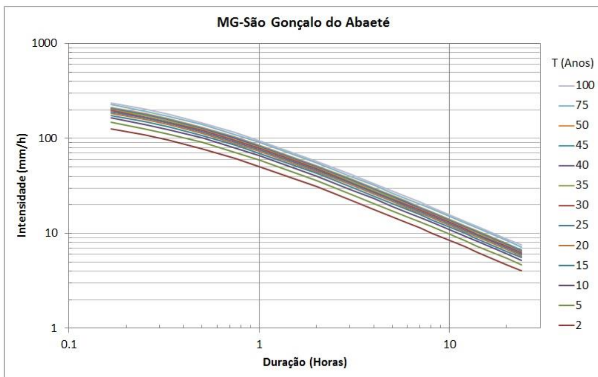
Figura 02 – Curvas intensidade-duração-frequência
