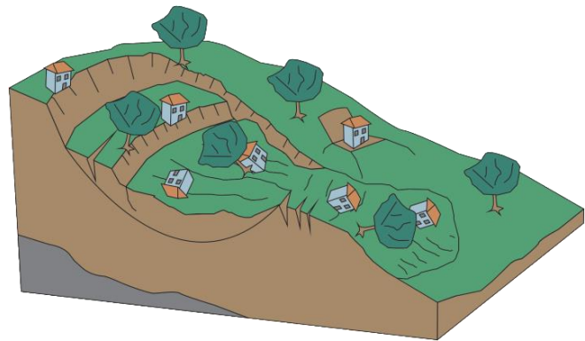
Figura 02 – Desenho esquemático de um deslizamento rotacional.
