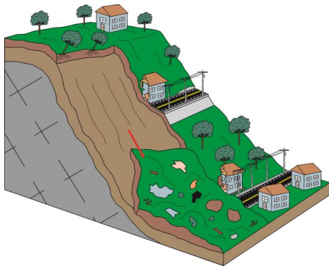
Figura 01 – Desenho esquemático de um deslizamento translacional.
