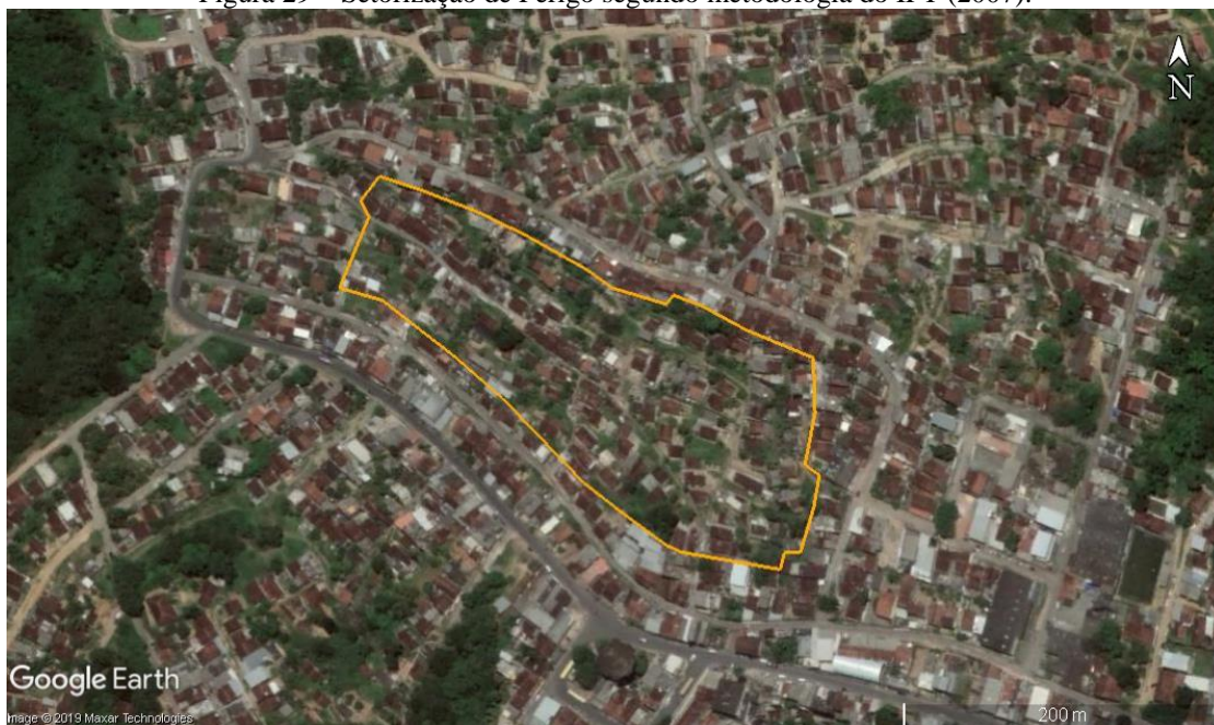
Figura 29 – Setorização de Perigo segundo metodologia do IPT (2007).
