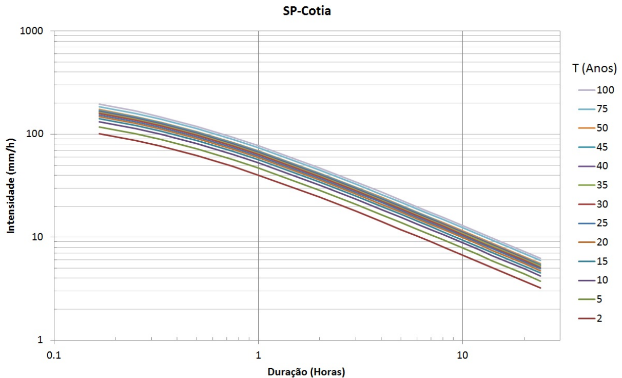
Figura 02 – Curvas intensidade-duração-frequência
