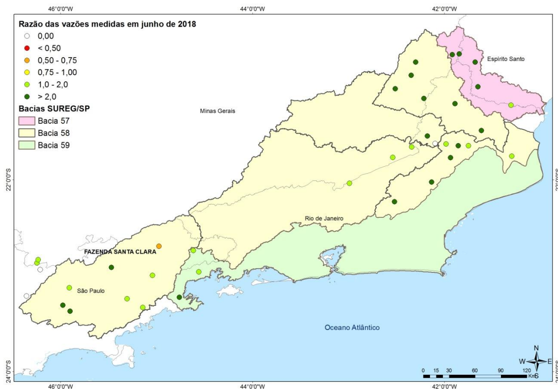
Figura 11 - Razão entre a vazão das medições de descarga líquida realizadas em junho de 2018 e a vazão mínima histórica medida até 2013
