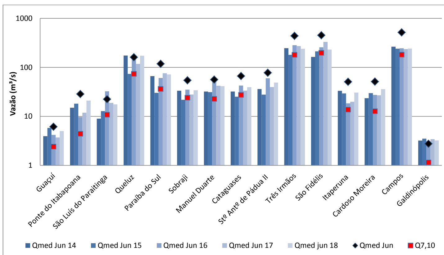
Figura 8 – Comparação entre a vazão média de junho de 2014, 2015, 2016, 2017 e 2018, média histórica de junho e vazão de referência Q_{7,10} nas estações indicadoras.
