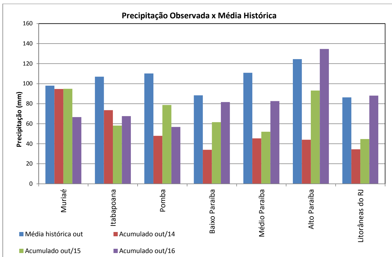
Figura 5 - Comparação entre a precipitação média histórica de outubro, e a precipitação acumulada de outubro de 2014, 2015 e 2016 nas bacias da área de atuação da SUREG/SP.
