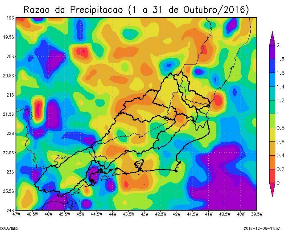
Figura 4 – Razão entre a precipitação acumulada no mês de outubro de 2016 e a média histórica de outubro (1998 a 2013).
