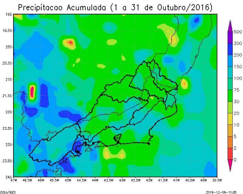
Figura 3 - Precipitação acumulada no mês de outubro de 2016.
