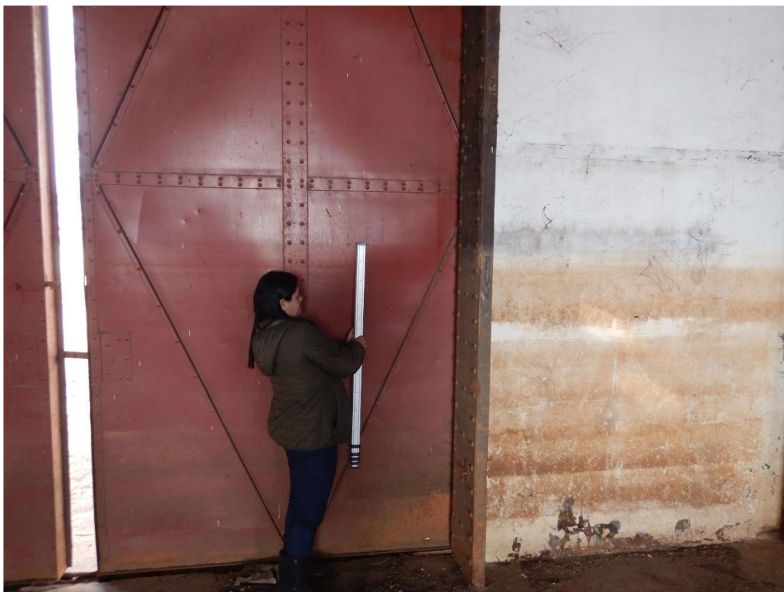
Figura 14: Nivelamento geométrico de marcas de cheia no Cais Mauá.
