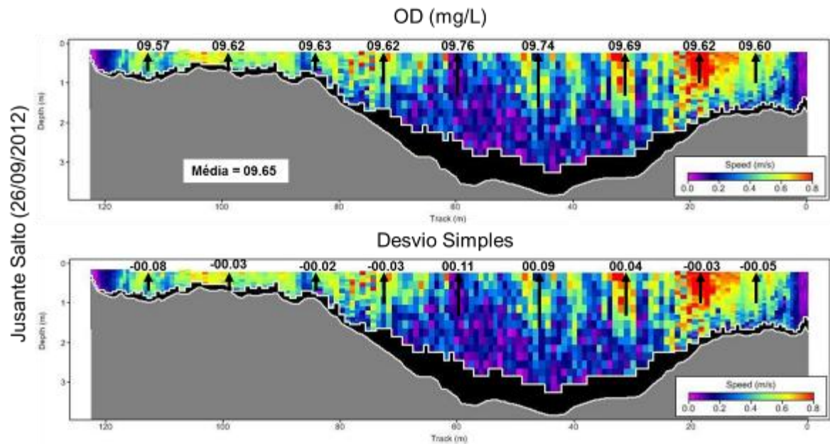
Figura 18 – Concentrações de OD na seção do ponto P09 no dia 26/09/2012.
