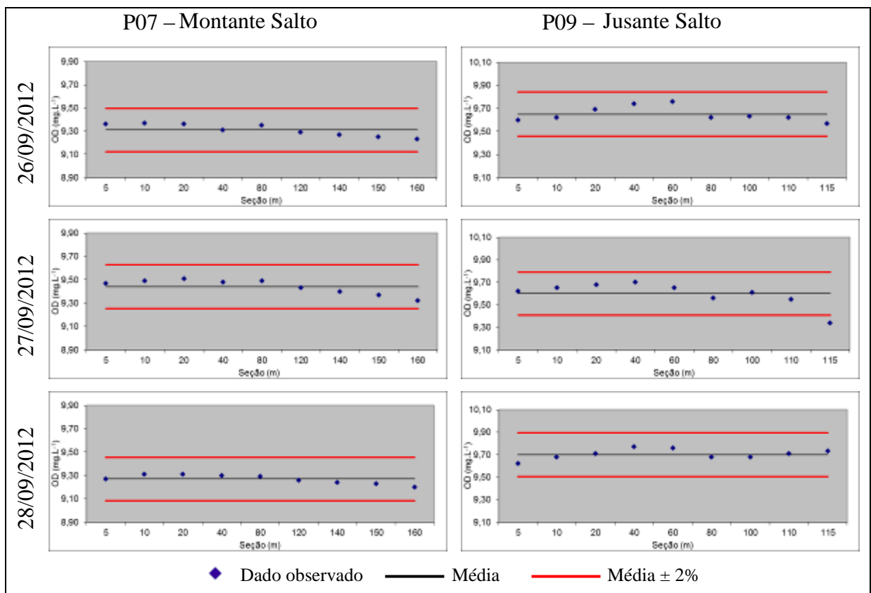
Figura 23 – Concentrações de OD na seção, média e faixa de \pm 2\% em relação à média.
