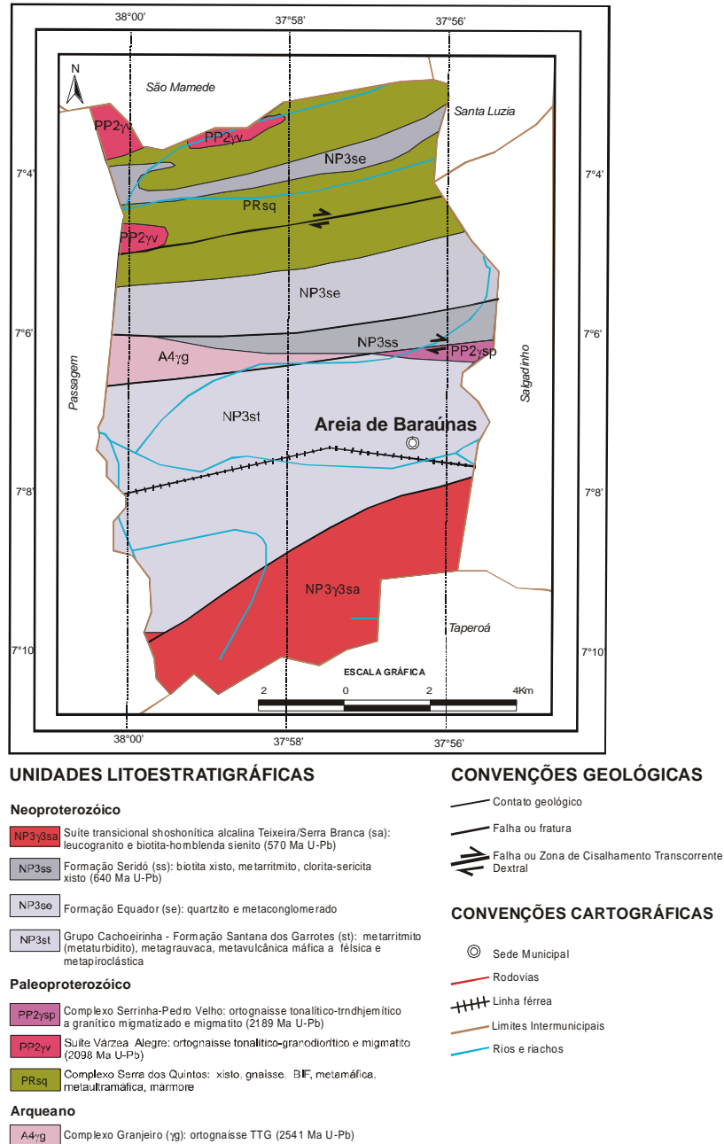
Figura 3 – Mapa Geológico
