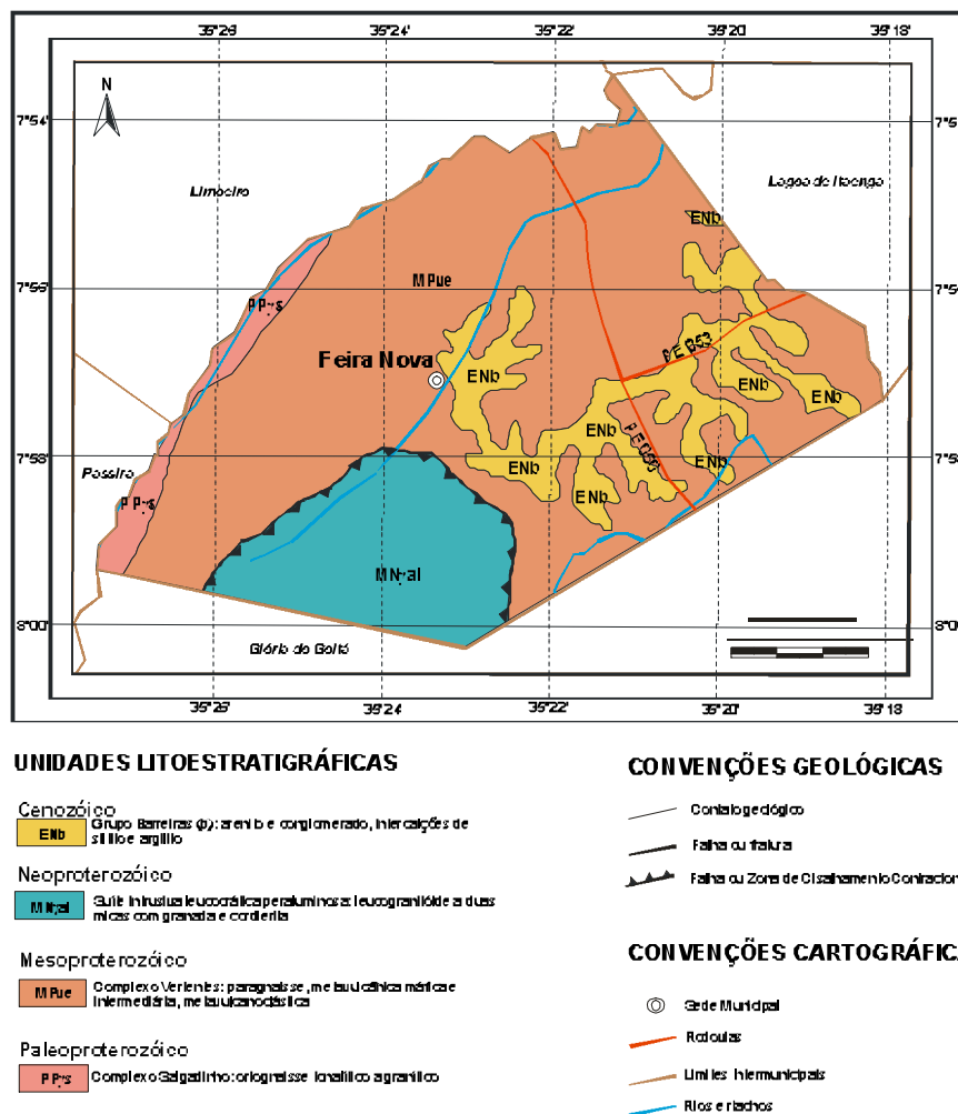
Figura 3 – Mapa Geológico
