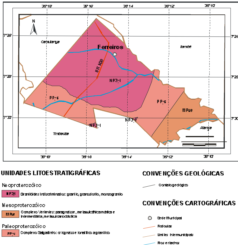
Figura 3 - Mapa Geológico
