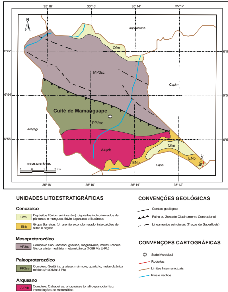
Figura 3 – Mapa Geológico
