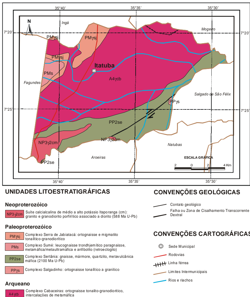
Figura 3 – Mapa Geológico
