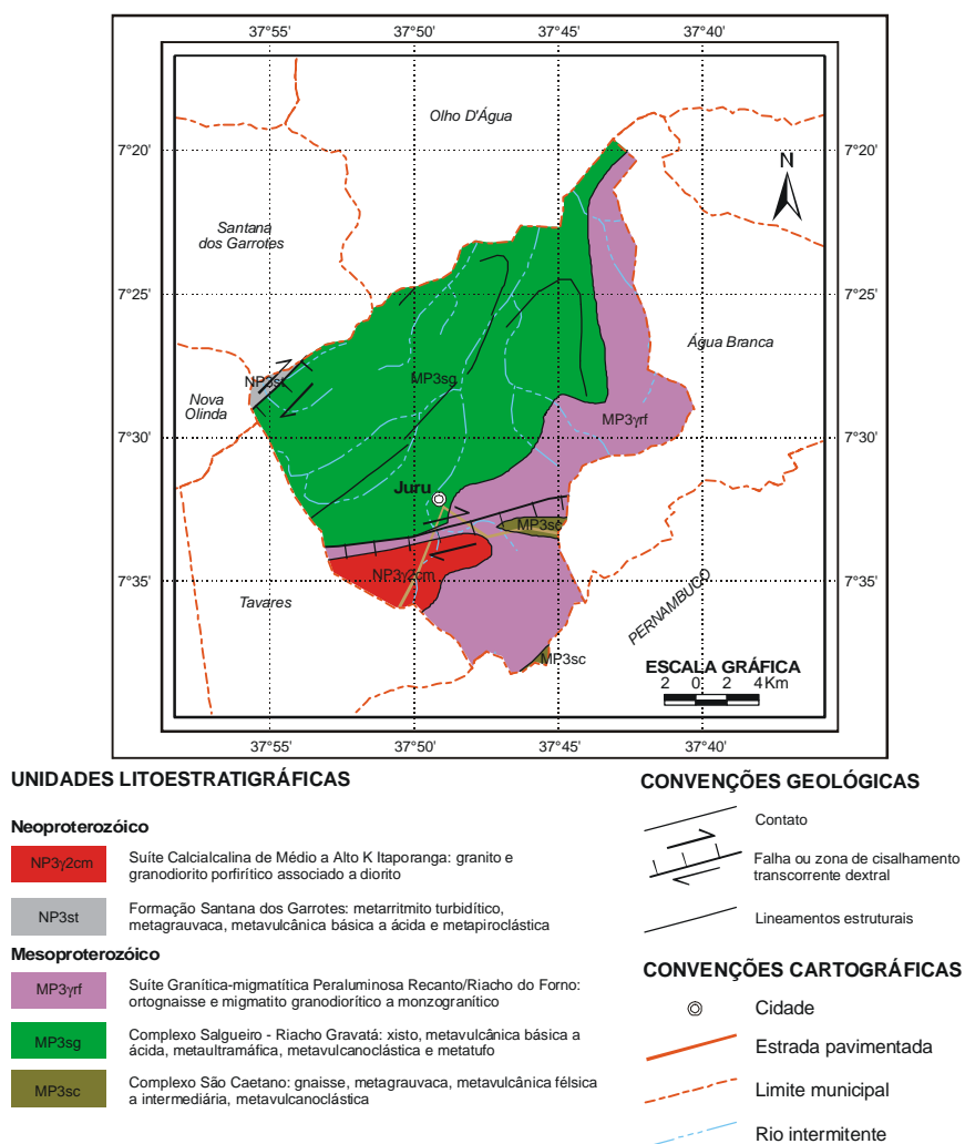
Figura 3 – Mapa Geológico
