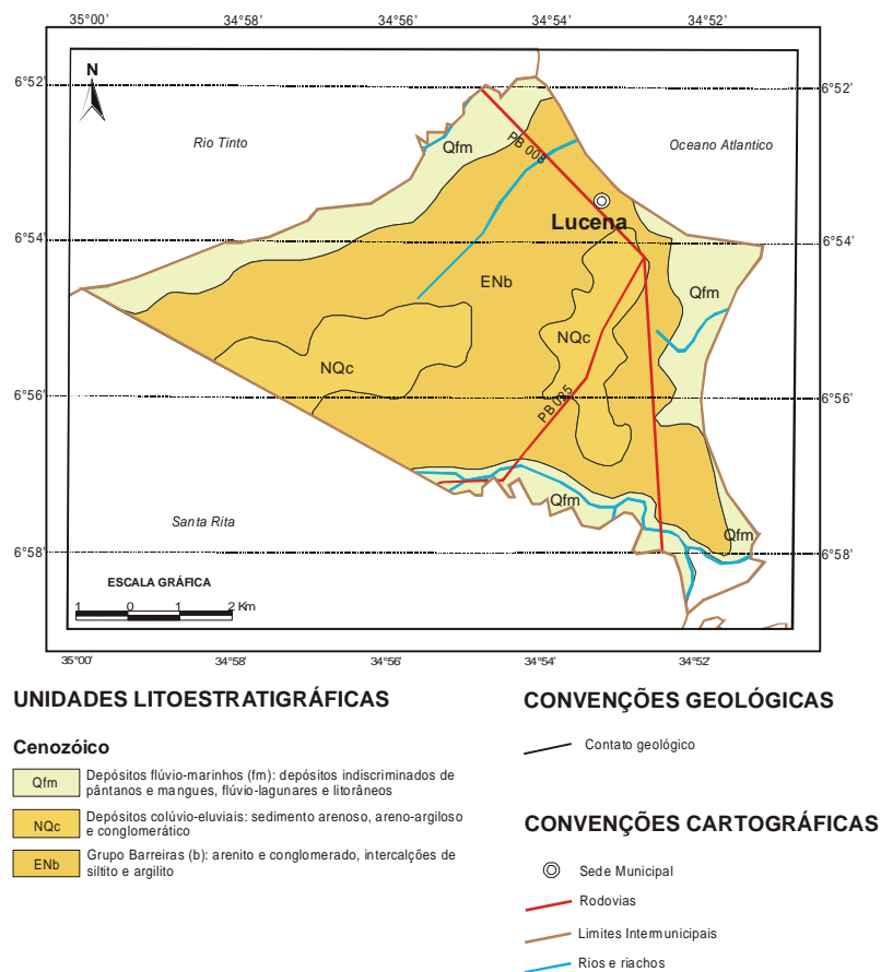
Figura 3 – Mapa Geológico
