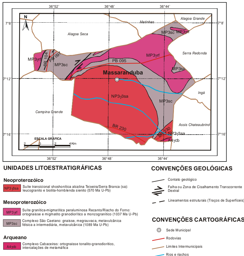
Figura 3 – Mapa Geológico
