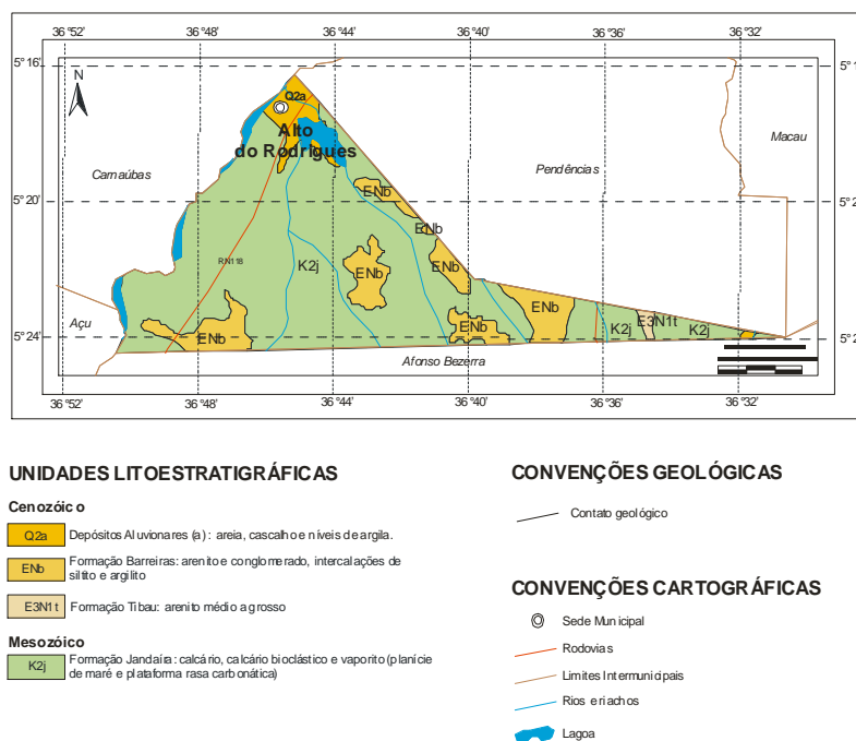
Figura 3 - Mapa Geológico
