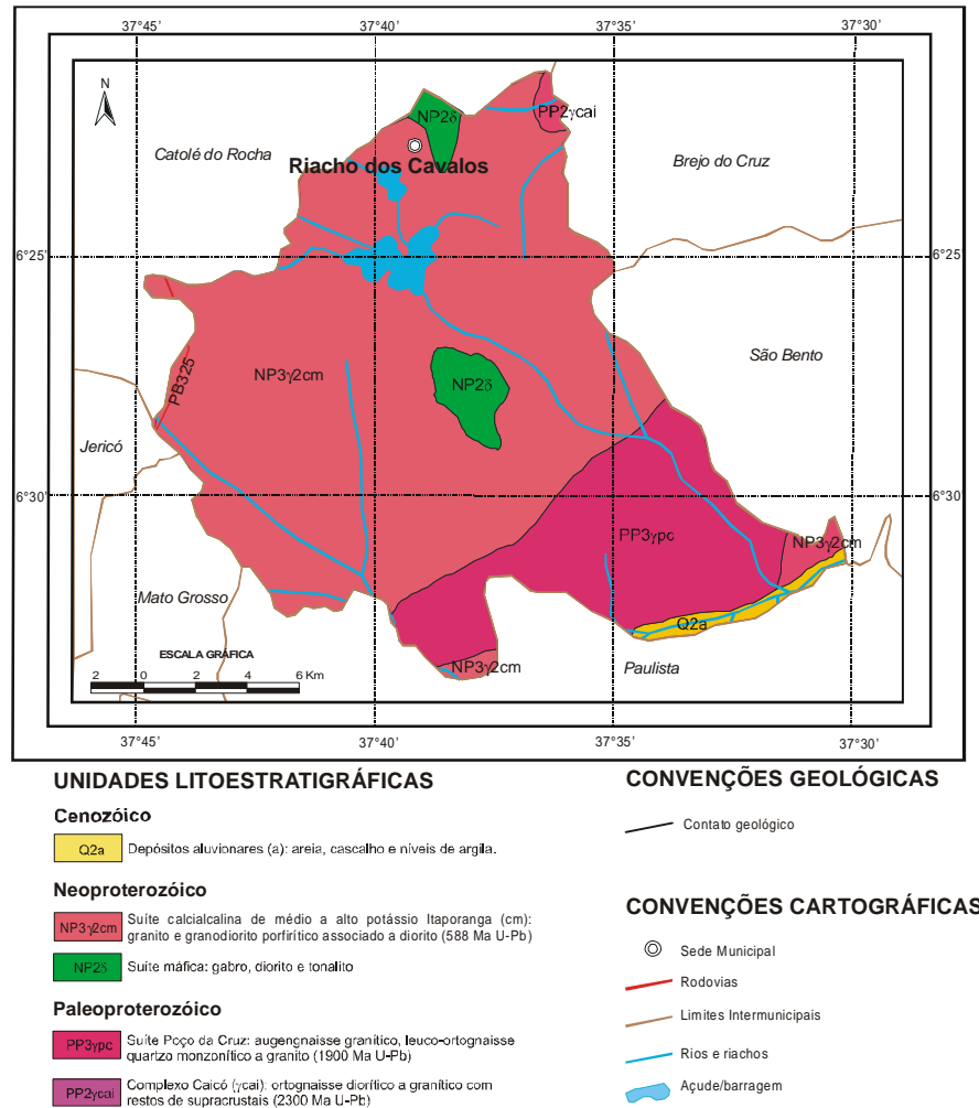
Figura 3 – Mapa Geológico
