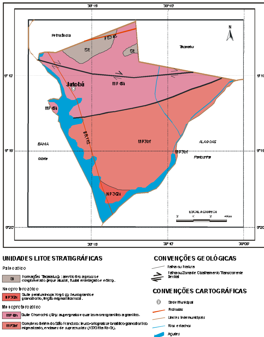
Figura 3 – Mapa Geológico
