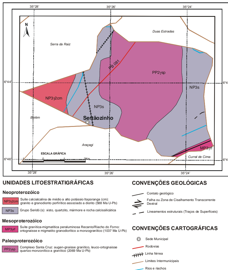
Figura 3 – Mapa Geológico
