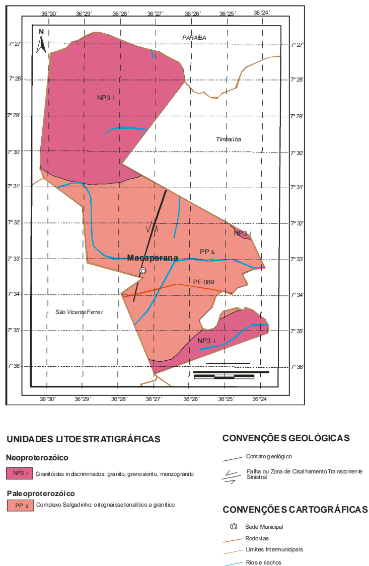
Figura 3 - Mapa Geológico
