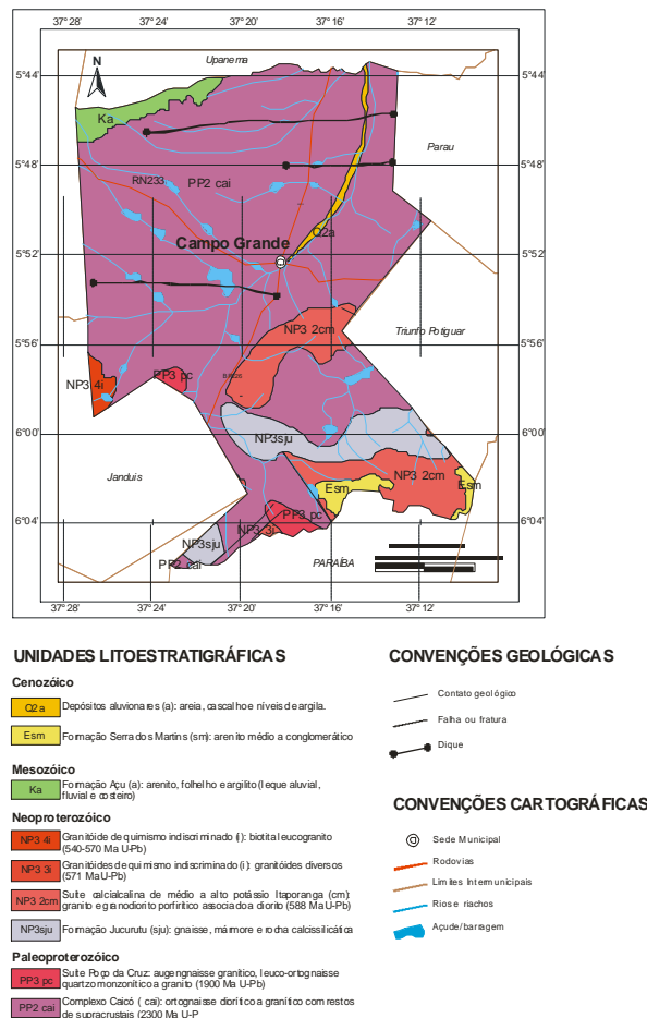
Figura 3 - Mapa Geológico
