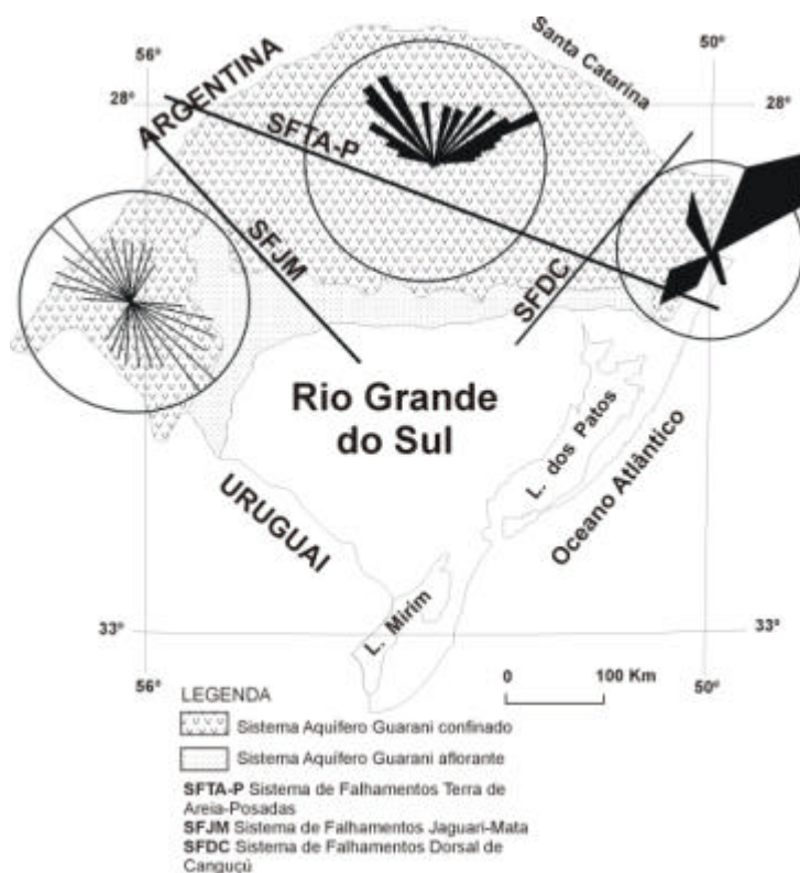
Figura 1 Principais sistemas de falhamentos que compartimentam o Sistema Aquífero Guarani no Rio Grande do Sul.
