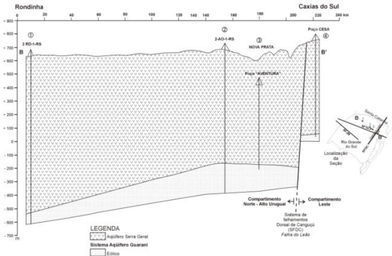
Figura 3 Seção geológica ilustrando o efeito do sistema de falhamentos da Dorsal de canguçu (SFDC) sobre o Sistema Aquífero Guarani, causando a elevação das cotas do topo do SAG no Compartimento Leste, em relação ao Compartimento Norte-Auto Uruguai.
