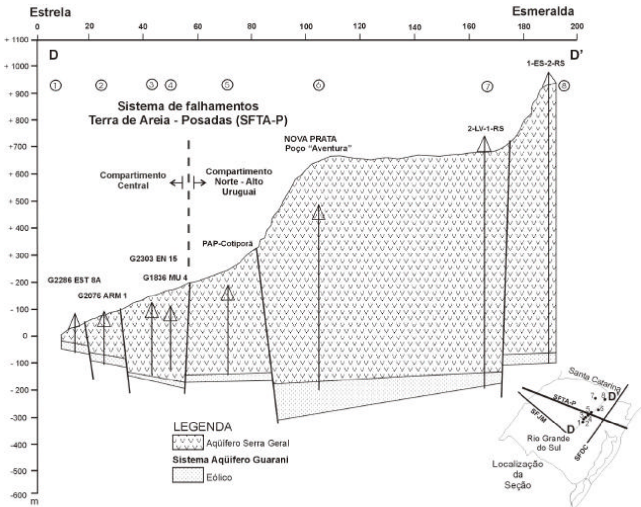
Figura 5 Seção Geológica onde visualiza-se o sistema de falhamentos Terra de Areia – Posadas delimitando os Compartimentos Central e Norte – Alto Uruguai.
