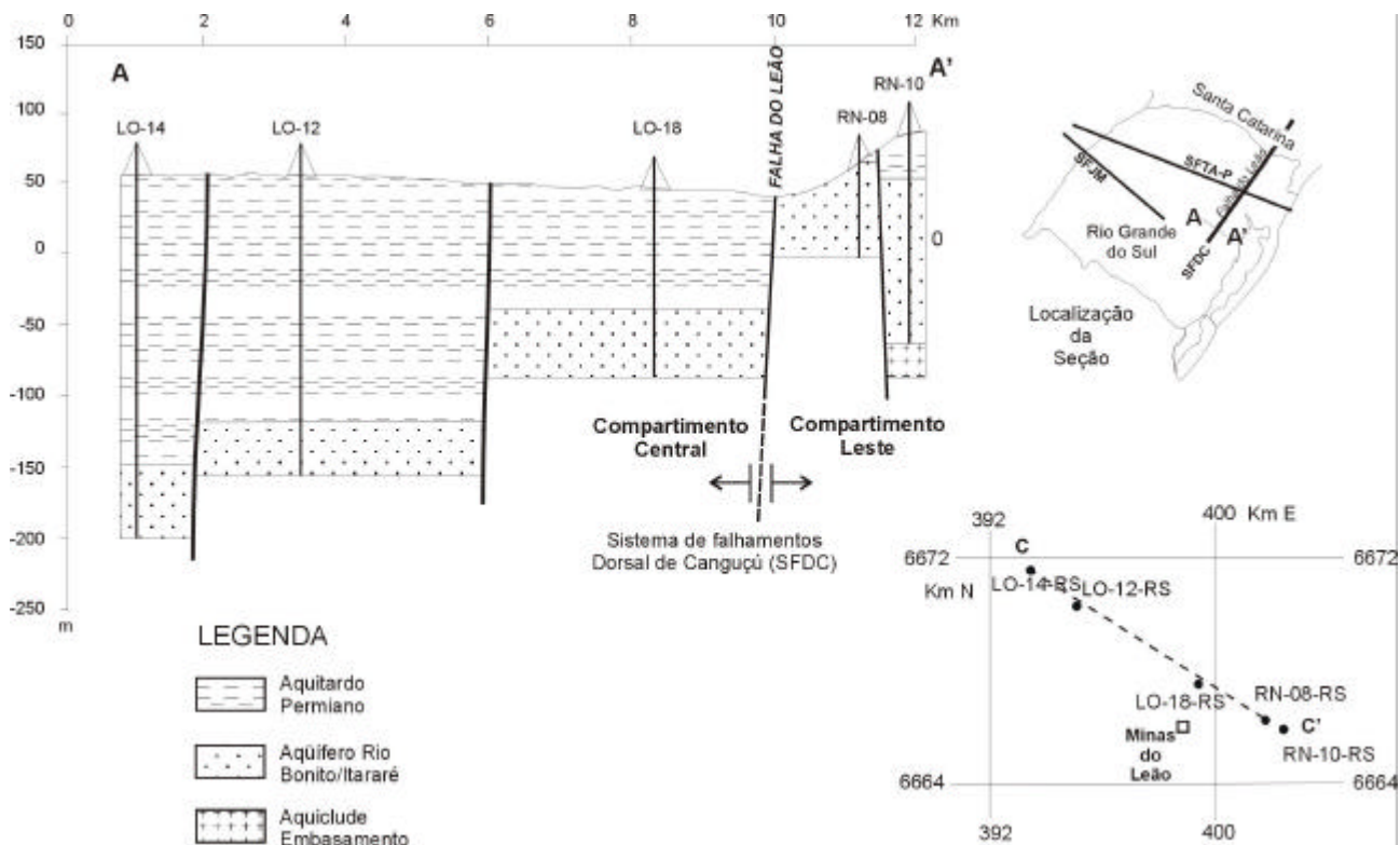
Figura 2 Seção geológica representando a compartimentação do Sistema Aquífero Guarani pelo sistema de falhamentos Dorsal de Canguçu (Falha do Leão).
