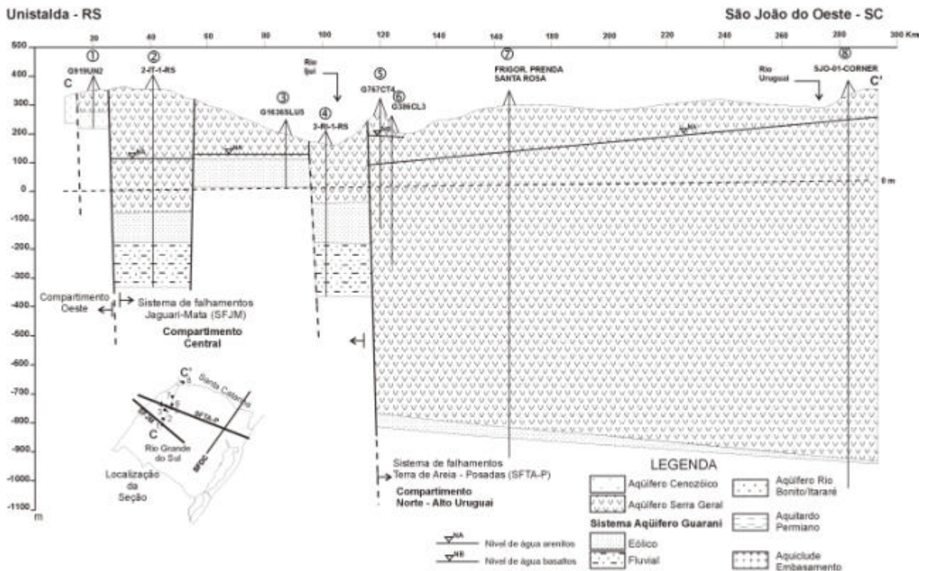
Figura 4 Seção hidrogeológica mostrando o sistema de falhamentos Jaguari-Mata (SFJM) delimitando os compartimentos Oeste e Central e O sistema de falhamentos Terra de Areia-Posadas (SFTA-P) que delimita os compartimentos Central e Norte-Alto Uruguai.
