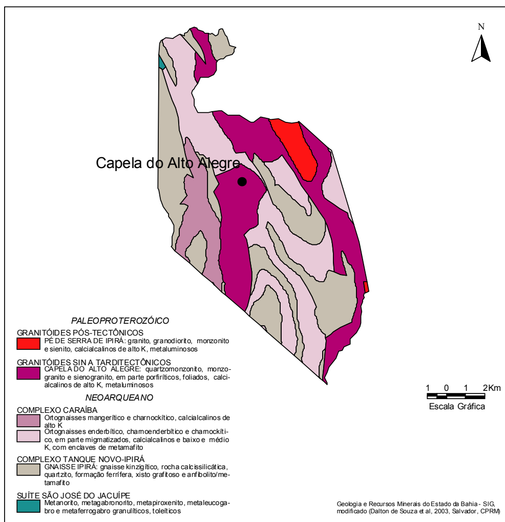
Figura 3 – Esboço geológico.
