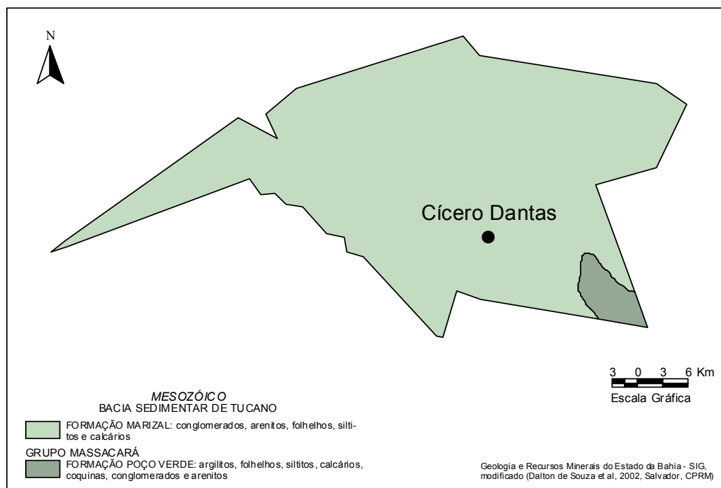
Figura 3 – Esboço geológico.
