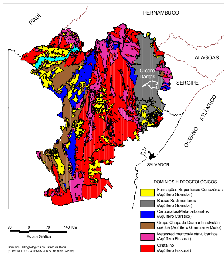
Figura 4 – Domínio hidrogeológico.
