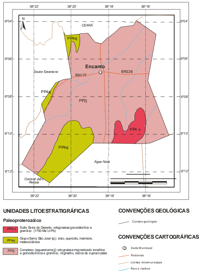
Figura 3 - Mapa Geológico
