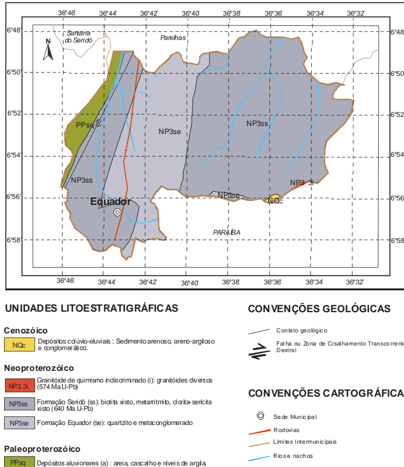
Figura 3 - Mapa Geológico
