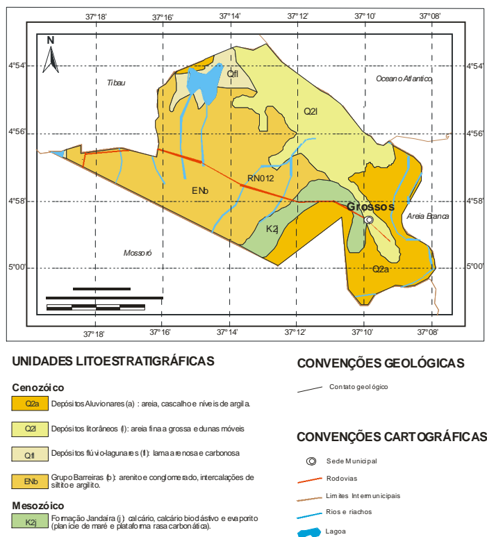
Figura 3 - Mapa Geológico
