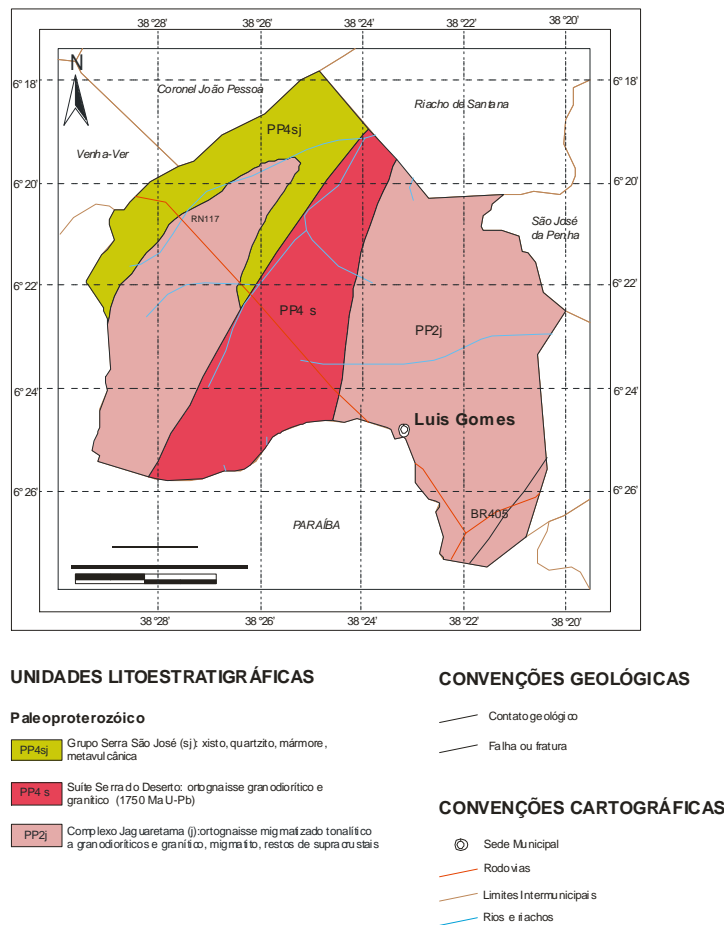
Figura 3 - Mapa Geológico
