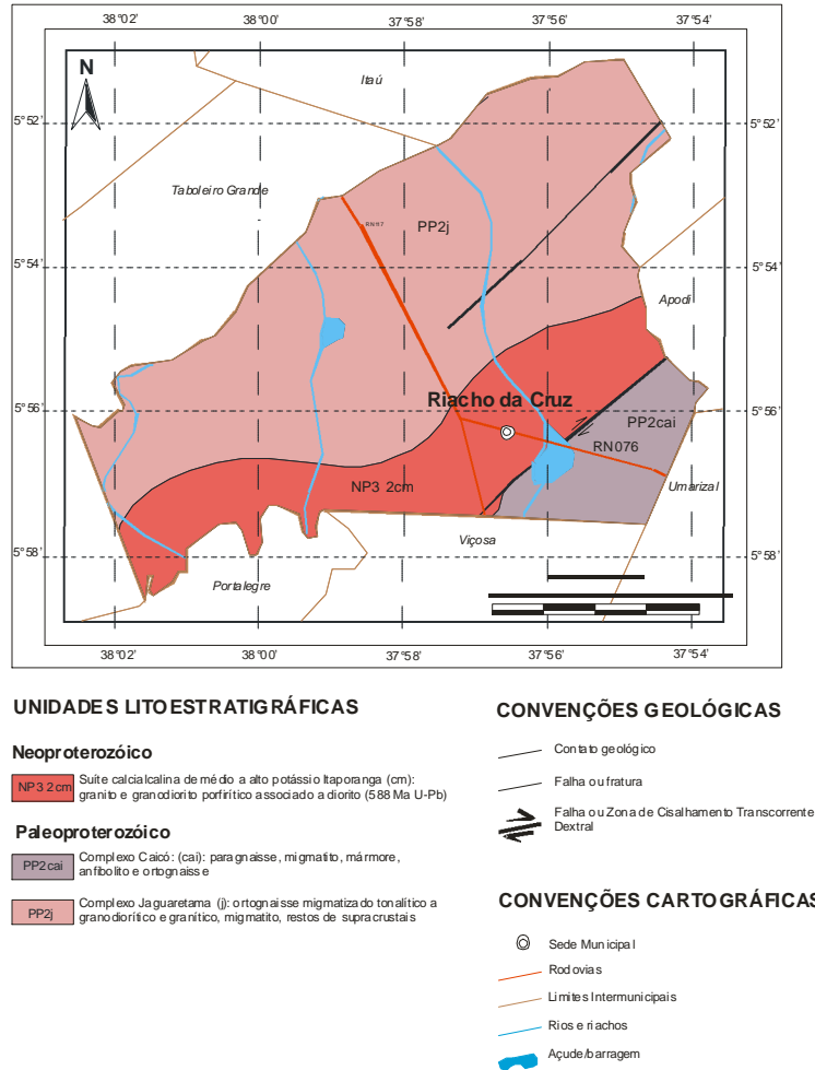
Figura 3 - Mapa Geológico
