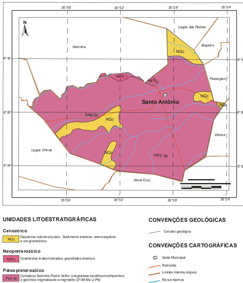
Figura 3 - Mapa Geológico
